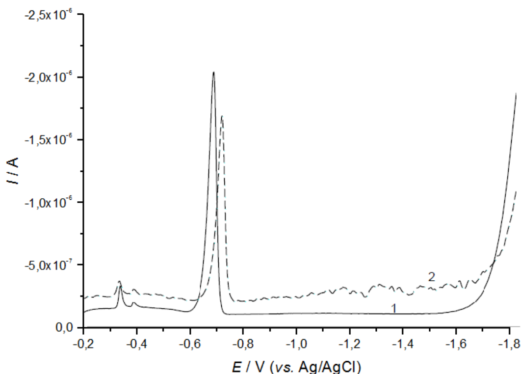
Slika 13. Linearna voltametrija u otopini \text{S}_5^{2-} 1 \times 10^{-7} \text{ mol dm}^{-3} prije zakiseljnja (krivulja 1) i nakon zakiseljenja i isplinjavanja strujom dušika (krivulja 2) u 0,55 \text{ mol dm}^{-3} \text{ NaCl} + 0,03 \text{ mol dm}^{-3} \text{ NaHCO}_3 ; E_d = -0,2 \text{ V} , t_d = 120 \text{ s} uz miješanje, v = 100 \text{ mV s}^{-1} (BAS elektroda)
