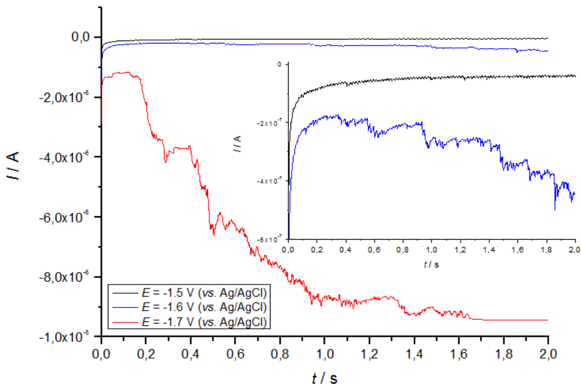
Slika 34. Kronoamperogrami snimljeni pri koncentraciji Fe 2+ i HS - od 5x10 -5 mol dm -3 u 0,091 mol dm -3 CaCl 2 pri E = -1,5 V (crna krivulja), E = -1,6 V (plava krivulja) i E = -1,7 V (crvena krivulja), t = 2 s uz t s = 0,0002 s; Umetak: krivulja snimljena na -1,5 V i -1,6 V s rasponom ordinate od -6x10 -7 do 0 A
