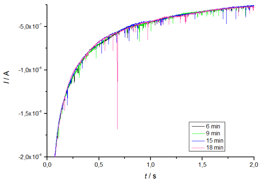
Slika 30. Kronoamperogrami snimljeni tijekom starenja disperzije sastava \text{Fe}^{2+} i \text{HS}^- koncentracije 5 \times 10^{-5} \text{ mol dm}^{-3} u 0,55 \text{ mol dm}^{-3} \text{ NaCl} , E = -1,9 \text{ V} t = 2 \text{ s} uz t_s = 0,0004 \text{ s}
