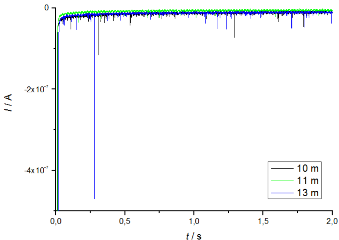
Slika 54. Kronoamperogrami snimljeni u uzorcima RJ prikupljenim 01/2016. koji su zakisljeni do \text{pH} = 2 i mjereni pri E = -0,8 V, t = 2 s uz t_s = 0,0004 s
