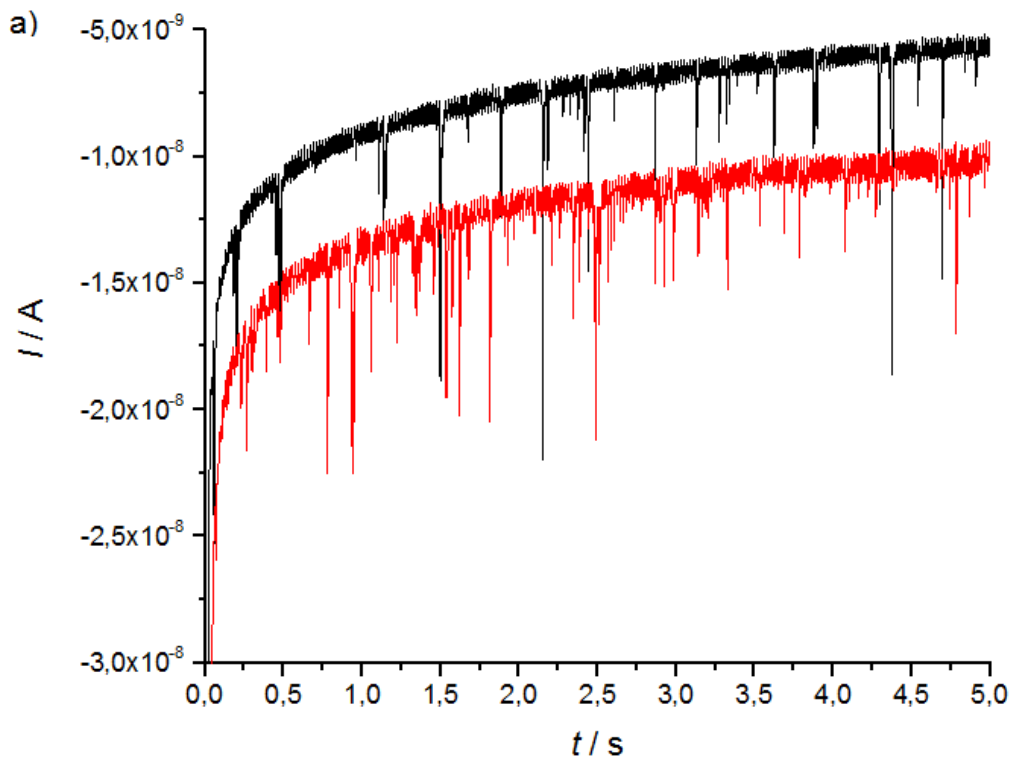
Slika 35. a) Kronoamperogrami snimljeni u disperziji \text{Ag}^+ koncentracije 6 \times 10^{-5} \text{ mol dm}^{-3} i \text{HS}^- koncentracije 3 \times 10^{-5} \text{ mol dm}^{-3} u 0,1 \text{ mol dm}^{-3} \text{NaCl} bez dodatka HA (crna krivulja) i uz dodatak HA koncentracije 5 \text{ mg dm}^{-3} (crvena krivulja); E = -1,2 \text{ V} , t = 2 \text{ s} uz t_s = 0,0004 \text{ s}
