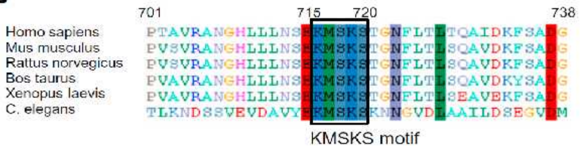
Slika 11. KMSKS motiv zajedni ko je svojstvo brojnih eukariota. Preuzeto iz [3].
