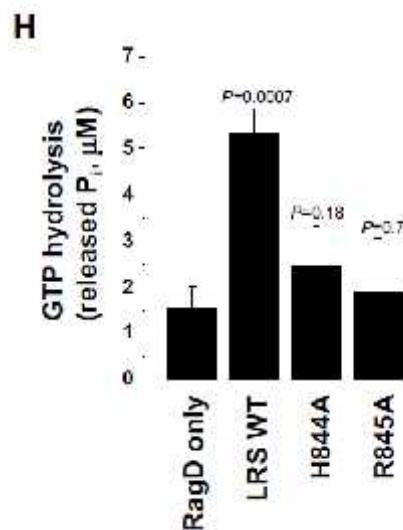
Slika 12. Utjecaj wt LRS i mutantnih LRS na hidrolizu GTP-a na RagD proteinu. Analize su vršene GTP-aznim analiznim kitom . Preuzeto iz [3].
