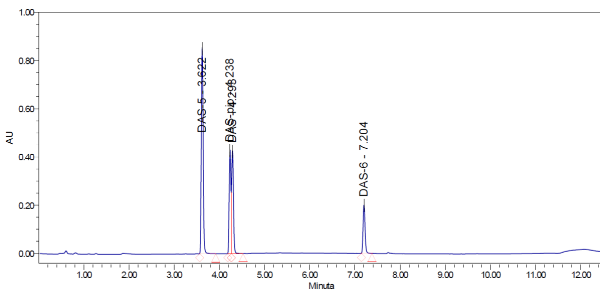
Slika D4. Kromatogram otopine dasatiniba i tri poznata onečišćenja analizirane na koloni Acquity UPLC CSH C18 1,7 \mu m; 2,1 mm \times 100 mm
