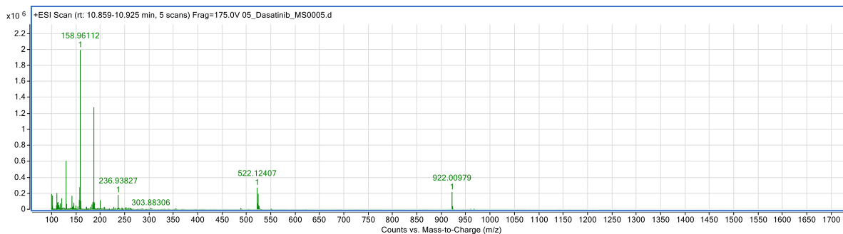
Slika D97. MS spektar uzorka dasatiniba koji tretiran s 1 mol dm -1 NaOH (pik pri ukupnom vremenu zadržavanja 10,859-10,925 min)
