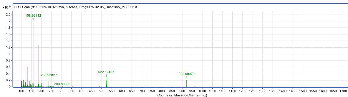
Slika D97. MS spektar uzorka dasatiniba koji tretiran s 1 \text{ mol dm}^{-1} NaOH (pik pri ukupnom vremenu zadržavanja 10,859-10,925 min)
