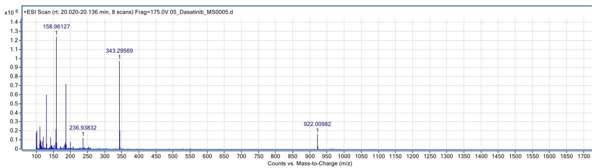
Slika D98. MS spektar uzorka dasatiniba koji tretiran s 1 \text{ mol dm}^{-1} NaOH (pik pri ukupnom vremenu zadržavanja 20,020-20,136 min)
