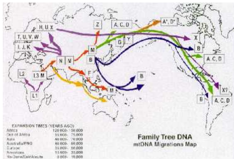
slika 1. Porijeklo ljudi prema mtDNA markerima
