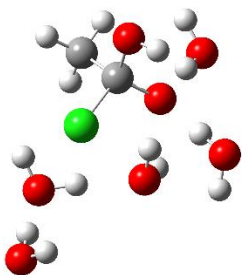
AcOHCl - -4 (0,45)
