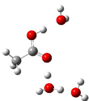
\text{AcOH}_2^+ -3-1 (0)
