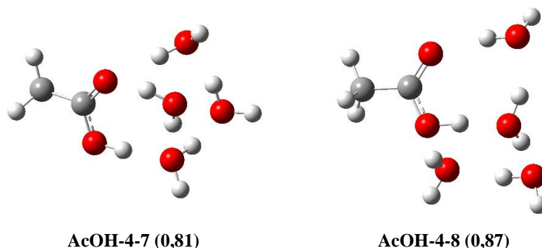
Slika 27. Geometrije AcOH s četiri molekule vode. Relativne energije, iskazane u kcal/mol, su naznačene u zagradama.
