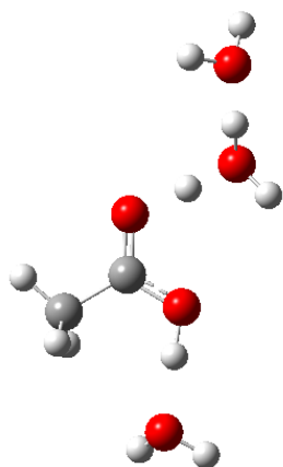
\text{AcOH}_2^+ -3-3 (0,12)
