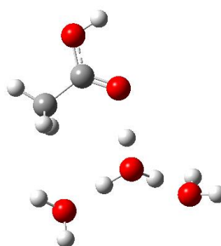
\text{AcOH}_2^+ -3-2 (0,03)
