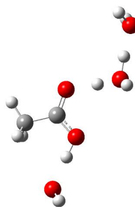
\text{AcOH}_2^+ -3-4 (0,39)
