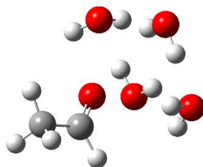
CH 3 CH=O-4-2 (0,18)
