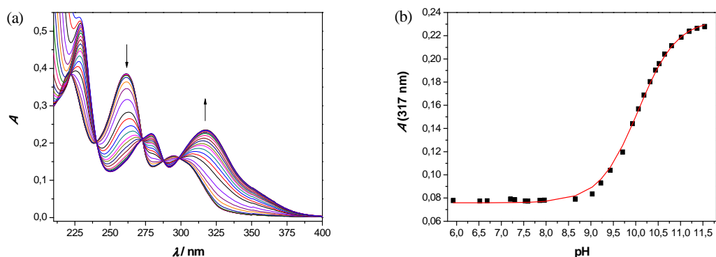
Slika 53. (a) Ovisnost apsorpcijskog spektra spoja 12 ( c = 9,5 \times 10^{-6} mol dm ^{-3} u CH _3 CN-H _2 O (3:7)) o pH (spektri su korigirani na razrjeđenje); (b) ovisnost apsorbanacije pri 317 nm o pH.
