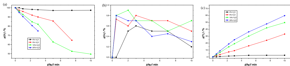
Slika 65. Ovisnost udjela pojedinih spoja o udjelu vode u metanolu i o vremenu ozračivanja za sol 19 . (a) Udio početnog spoja 19 ; (b) udio produkta fotohidrolize 14 ; (c) udio produkta fotometanolize 71 .
