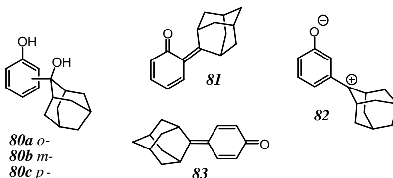
Slika 13. Strukture hidroksibenzilnih alkohola 80a-c i odgovarajućih QM 81-83 s adamantanskim supstuentom. 19
