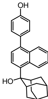
Prilog 32. ^1\text{H} NMR (300 MHz, \text{CDCl}_3 ) i ^{13}\text{C} NMR (75 MHz, \text{DMSO-d}_6 ) spektri ( \delta/\text{ppm} ) 4-(2-hidroksi-2-adamantil)-1-(4-hidroksifenil)naftalena ( 8 ).
