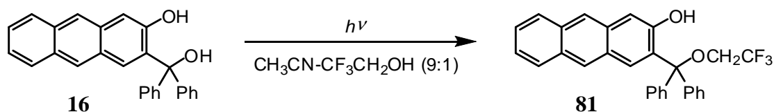
Shema 71. Fotokemija spoja 16 u prisutnosti 2,2,2-trifluoetanol.
