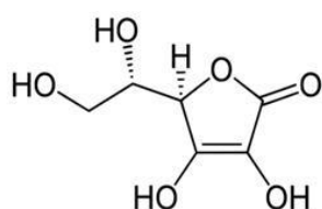
AscH
