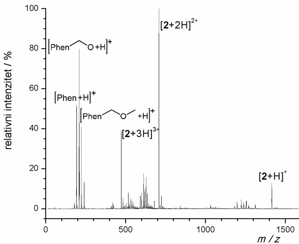
Slika 44. Maseni spektar spoja 2 u smjesi otapala MeCN/CH 2 Cl 2 ( \phi = 0,5 ) nakon ozračivanja u fotokemijskom reaktoru.
