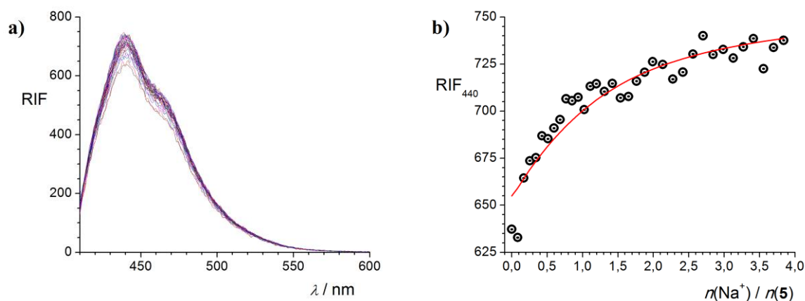
Slika 110. a) Fluorimetrijska titracija spoja 5 ( c = 7,2 \times 10^{-7}\text{ mol dm}^{-3} ) s NaClO 4 ( c = 5,121 \times 10^{-5}\text{ mol dm}^{-3} ) u smjesi otapala MeOH/CH 2 Cl 2 ( \varphi = 0,5 ); \vartheta = (25,0 \pm 0,1)^\circ\text{C} ; V_0(5) = 2,5\text{ cm}^3 ; \lambda_{\text{ex}} = 404\text{ nm} ; širine pukotina: ulazna 5 nm, izlazna 2,5 nm; l = 1\text{ cm} . Spektri su korigirani za razrjeđenje. b) Ovisnost relativnog intenziteta fluorescencije otopine spoja 5 pri 440 nm o omjeru množina dodanog NaClO 4 i spoja 5. \circ eksperimentalne vrijednosti; — izračunane vrijednosti.
