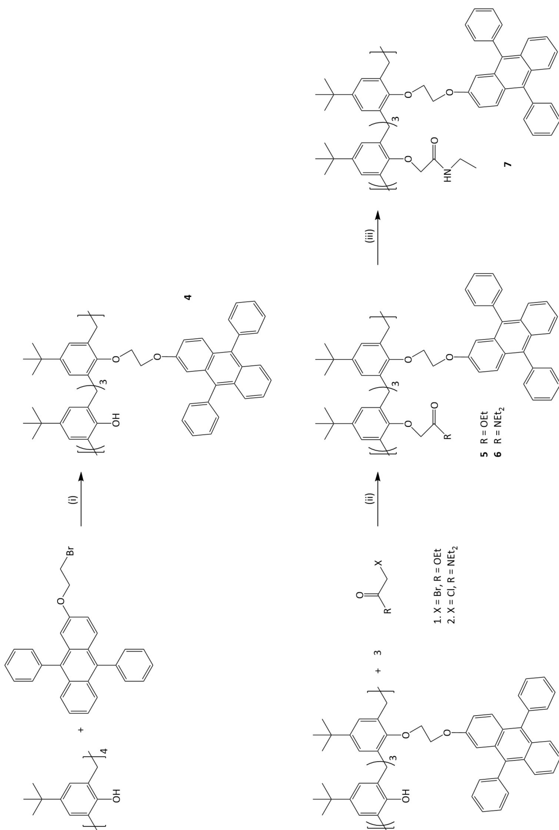
Shema 5. Priprava difenilantracenskih derivata kaliks[4]arena 4 , 5 , 6 i 7 . Reagensi i reakcijski uvjeti: (i) 1) K 2 CO 3 , KI, MeCN (Ar) Δ; (ii) 1) K 2 CO 3 , KI, acetone (Ar), Δ; (iii) etilamin.
