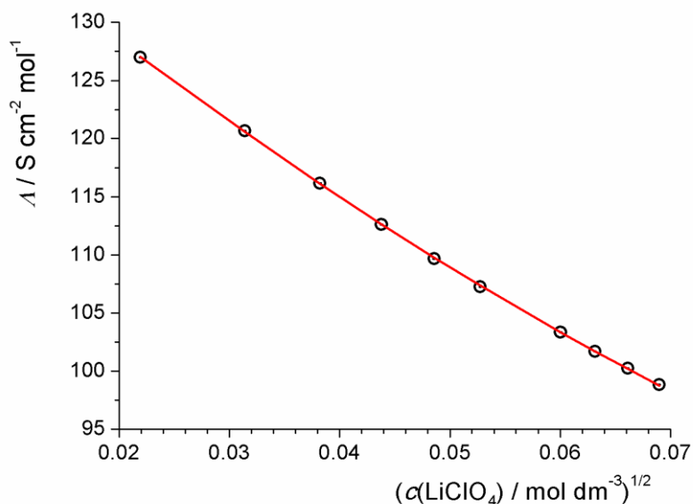
Slika 27. Ovisnost molarne provodnosti LiClO 4 o njegovoj koncentraciji u smjesi otapala MeCN/CH 2 Cl 2 ( \varphi = 0,5 ); \vartheta = (25,0 \pm 0,1) ^\circ\text{C} .
