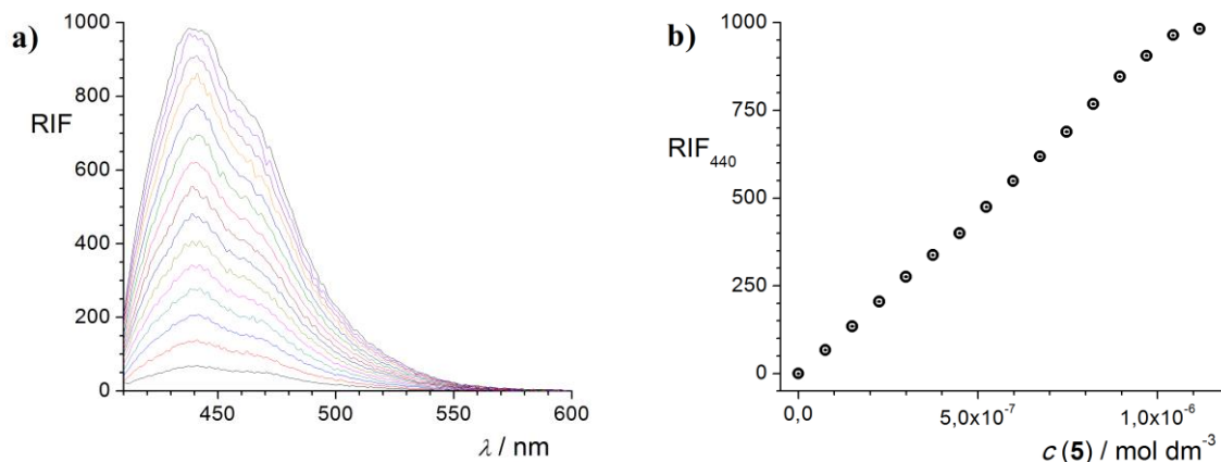
Slika 109. a) Ovisnost emisijskih spektara spoja 5 u smjesi otapala MeOH/CH 2 Cl 2 ( \varphi = 0,5 ) o njegovoj koncentraciji; \vartheta = (25,0 \pm 0,1)^\circ\text{C} ; V_0 = 2,5\text{ cm}^3 ; \lambda_{\text{ex}} = 404\text{ nm} ; širine pukotina: ulazna 5 nm, izlazna 2,5 nm; l = 1\text{ cm} . b) Ovisnost relativnog intenziteta fluorescencije otopine spoja 5 pri 440 nm o njegovoj koncentraciji.
