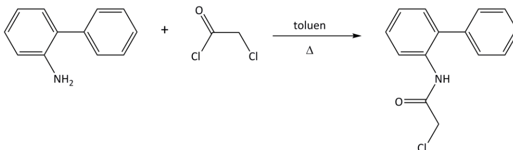
Shema 1. Sinteza 2-(kloracetamido)bifenila.
