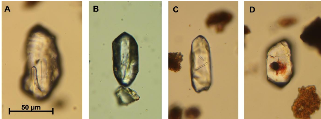
Slika 4.8: Uklopoci u kristalima cirkona: (A) cirkon; (B) fluidne inkluzije?; (C) apatit; (D) hematit. Snimljeno optičkim mikroskopom, N-.
