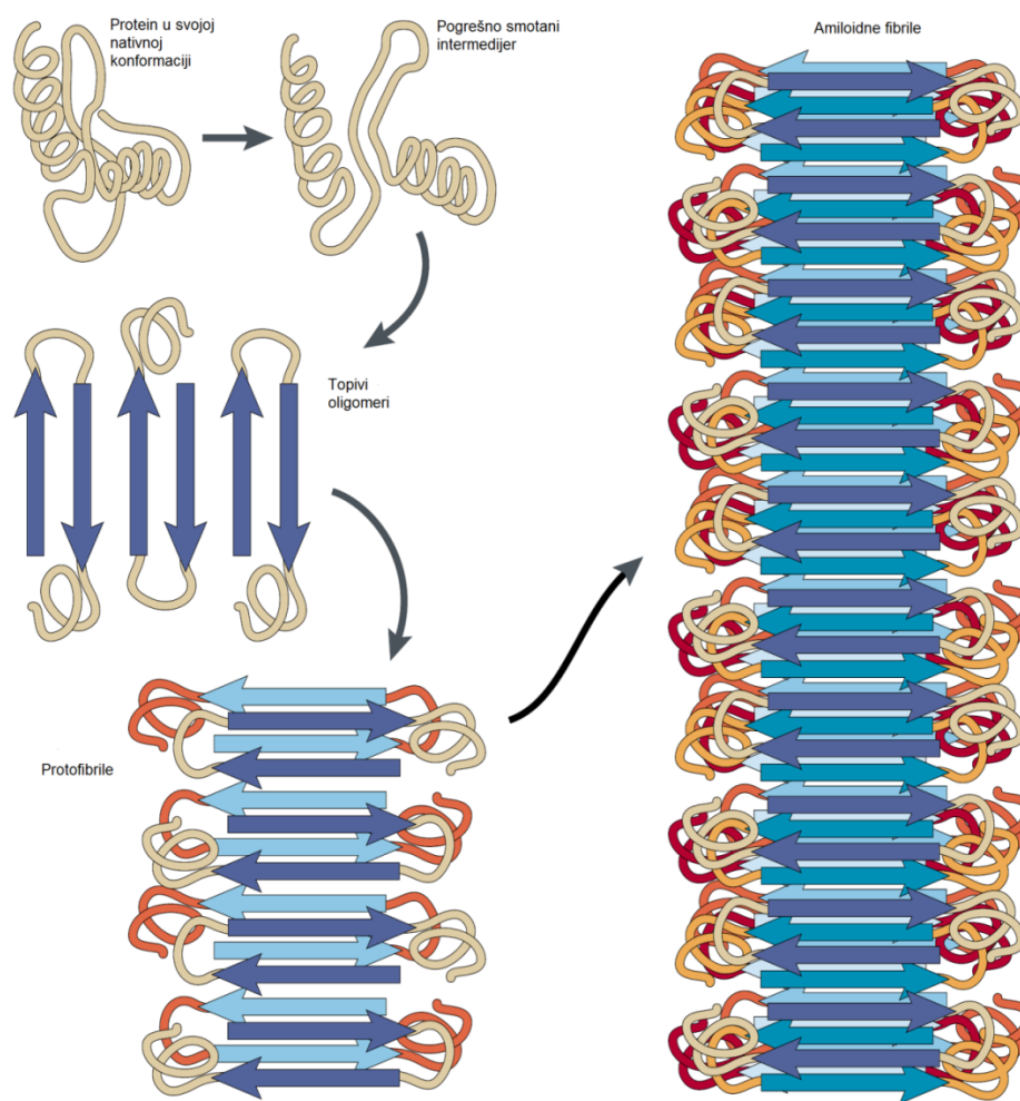
Slika 1. Shematski prikaz postupne agregacije pogrešno smotanih proteina u amiloidne agregate u obliku fibrilarnih niti (Soto, 2003).
