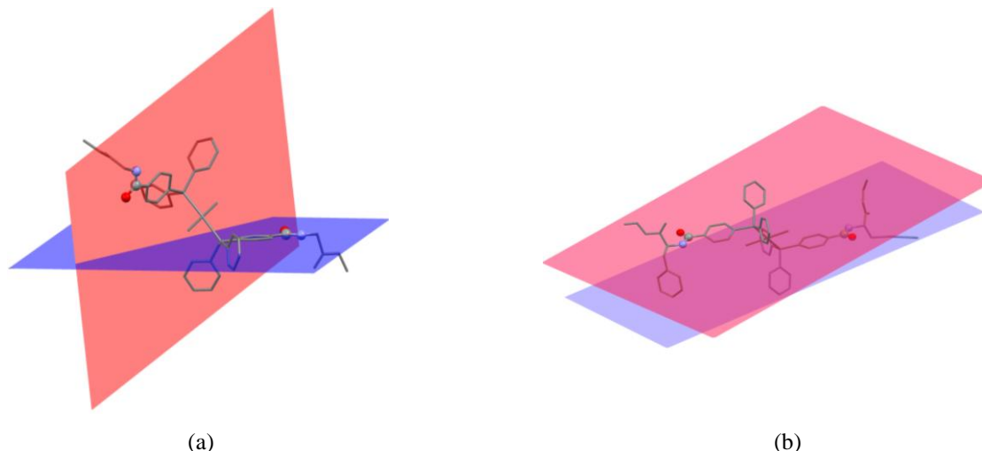
Slika 71. Ravnine u kojima leže amidne veze liganda u \text{trans}-[\text{PdCl}_2(\mathbf{L})_2] s ligandima (a) \mathbf{A1a} i (b) \mathbf{A1m} , zatvaraju kutove od 69^\circ odnosno 8^\circ .
