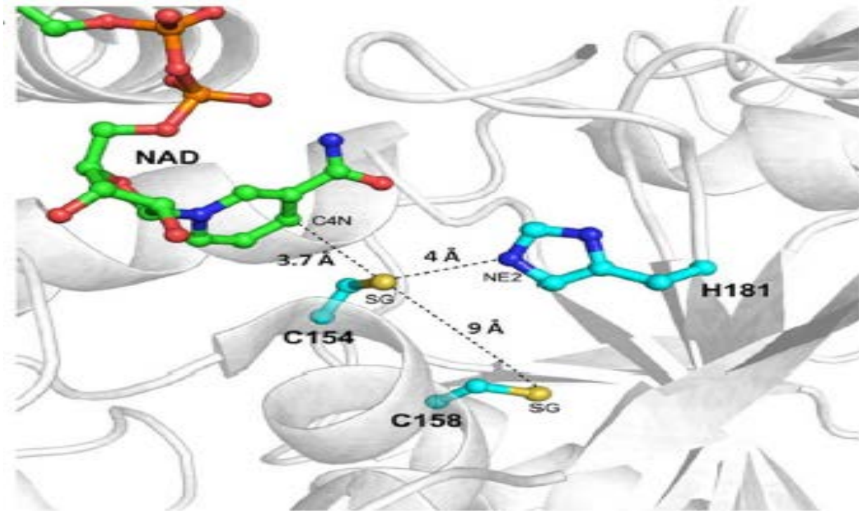
Slika 1.: Kristalna struktura katalitičkog mjesta citoplazmatske GAPDH iz riže ( Oryza sativa ) sa vezanim kofaktorom \text{NAD}^+ . Bojom su posebno istaknuti bočni ogranci Cys-154 i His-181 koji su bitni za katalizu te bočni ogranak Cys-158. (preuzeto iz Zaffagnini i sur. 2013)
