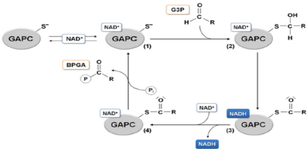
Slika 2.: Shematski prikaz reakcijskog mehanizma biljne citoplazmatske GAPDH (GAPC). 1) Supstrat (G3P) se veže u aktivno mjesto enzima, ali samo ako je kofaktor NAD^+ prisutan. 2) Deprotonirani bočni ogranak Cys-154 nukleofilno napada karbonilnu skupinu G3P i nastaje hemitioacetalni intermedijer. 3) Dolazi do oksidacije, H^+ sa intermedijera se prenosi na NAD^+ koji se reducira u NADH i otpušta sa enzima. Nastane novi acil-enzim intermedijer. 4) NAD^+ se veže u svoje mjesto na GAPDH. Anorganski fosfat reagira sa acil-enzim intermedijerom i otpušta se produkt (BPGA). (preuzeto iz Zaffagnini i sur. 2013)
