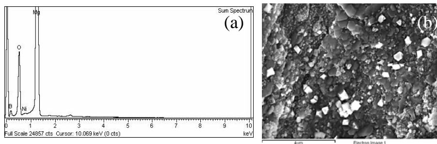
Slika 7.50. Zbirni EDS spektar uzorka MgB_2+Ni/C , 2,5 mas.%, (a) uzet s dijela uzorka prikazanog na slici (b) s mjernom ljestvicom od 4 µm.
