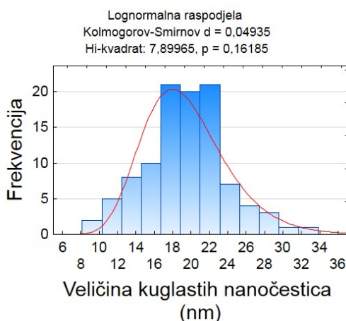
Slika 7.49. Raspodjela veličine kuglastih nanočestica u uzorku MgB 2 +Ni/C, 10 mas.%.
