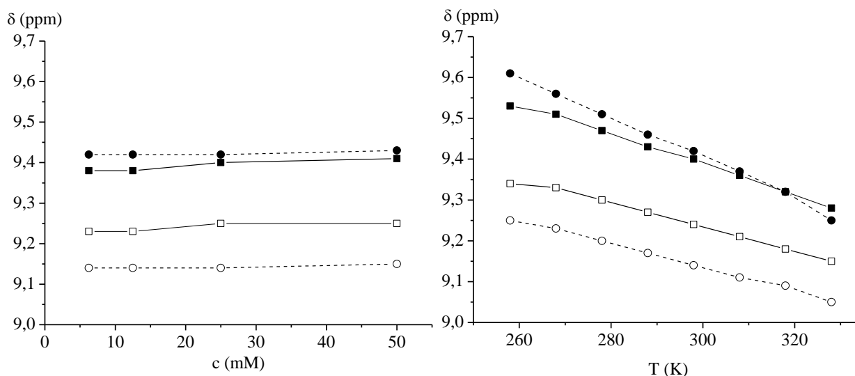
Slika 70. Koncentracijska-[ lijevo ; 21 ■(NH 1 F n ), □(NH 2 F n ); 22 ●(NH 1 F n ), ○(NH 2 F n )] i temperaturna-ovisnost amidnih protona tripeptida 21 i 22 [ desno ; 21 ■(NH 1 F n ), □(NH 2 F n ); 22 ●(NH 1 F n ), ○(NH 2 F n )]
