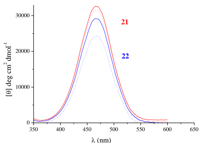
Slika 73. CD-spektri dipeptida 21 i 22 u CH 2 Cl 2 [ c = 5 \times 10^{-3} \text{M} (puna crta)] i uz dodatak 20 % DMSO (isprekidana crta)
