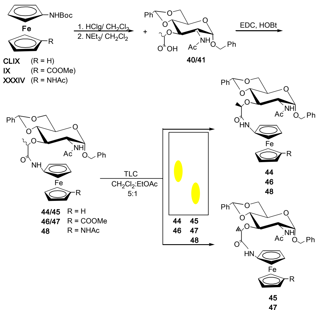
Shema 30. Sintaza ferocenskih muopeptida 44-48
