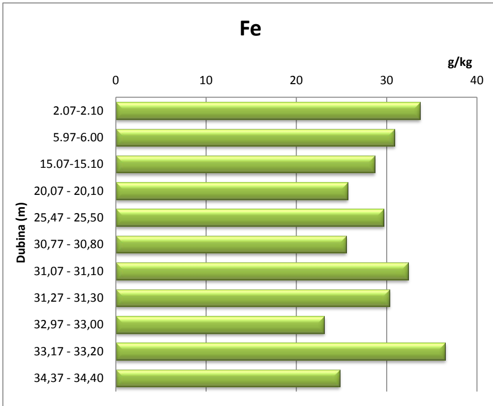
Slika 43. Koncentracija željeza
