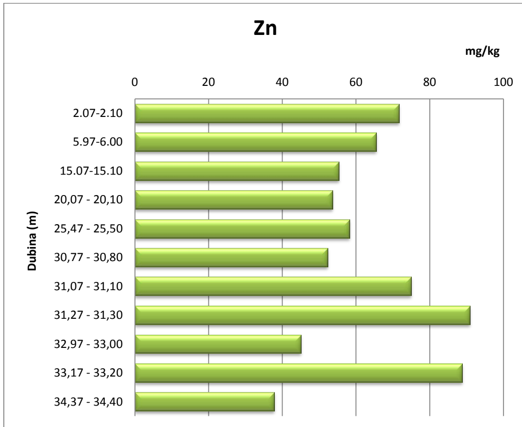
Slika 54. Koncentracija cinka
