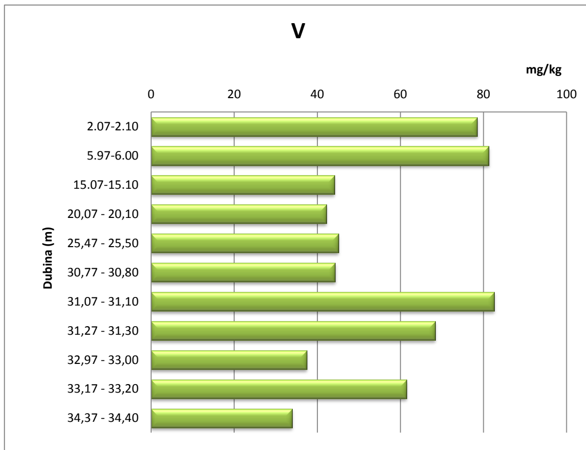
Slika 59. Koncentracija vanadija
