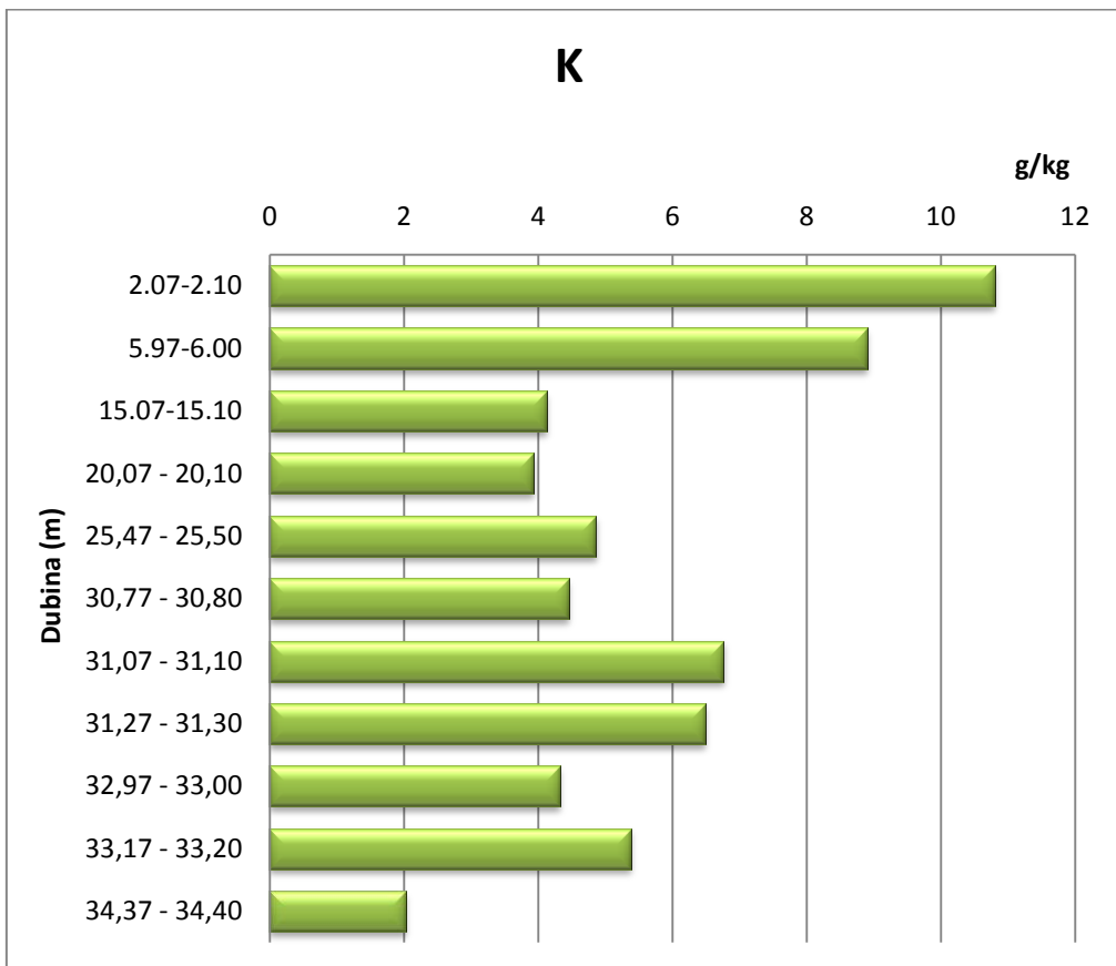
Slika 44. Koncentracija kalija
