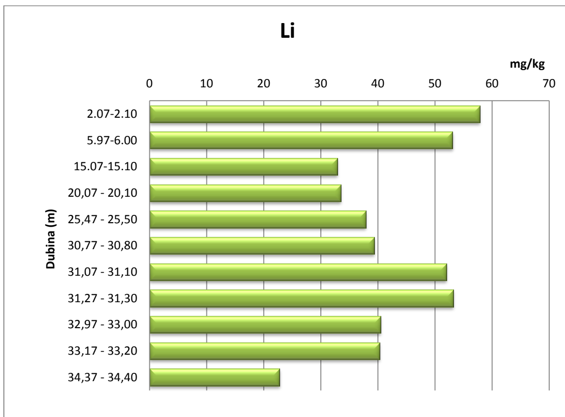
Slika 62. Koncentracija litija
