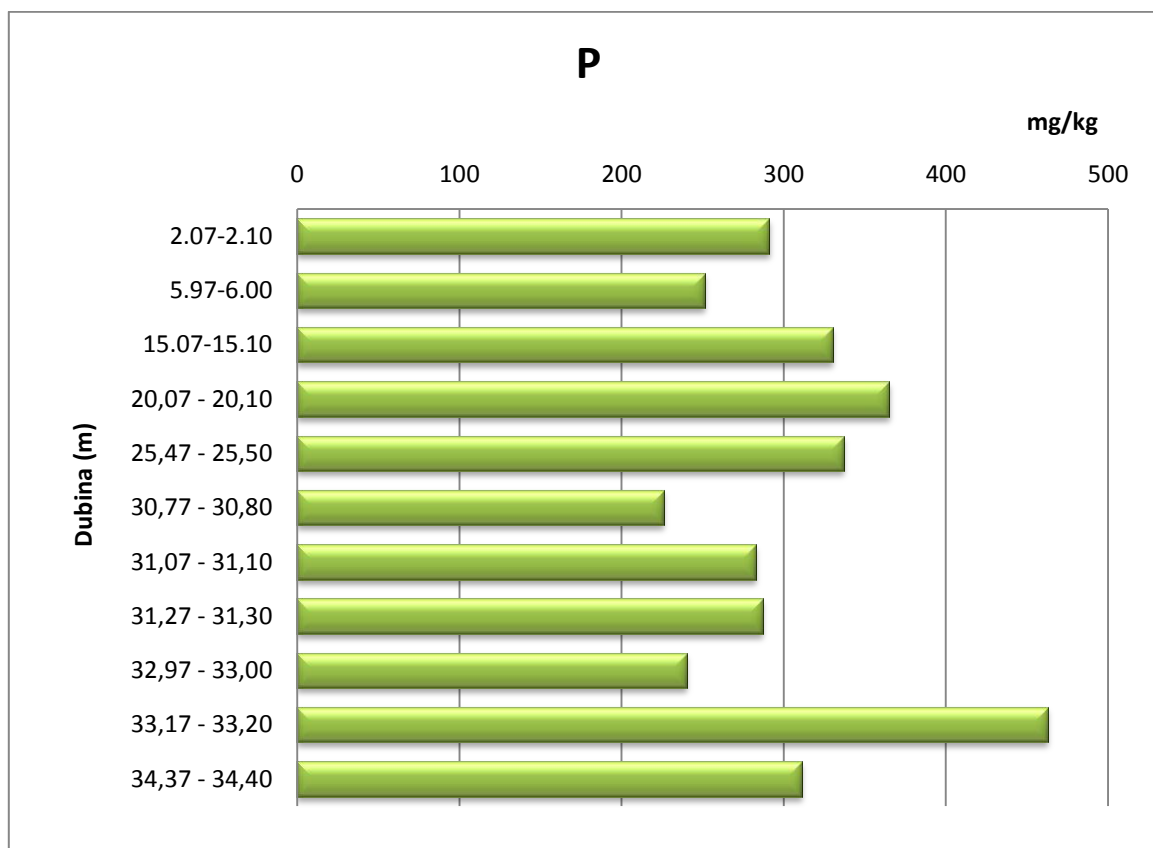
Slika 56. Koncentracija fosfora
