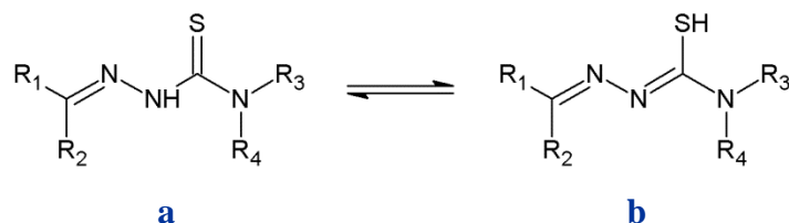
Slika 2-3. Tautomerni oblici tiosemikarbazona: a) tionski, b) tiolni.
