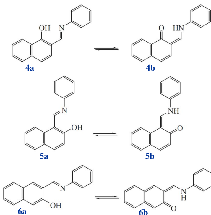
Slika 2-10. Strukture tautomera Schiffovih baza 4–6 .
