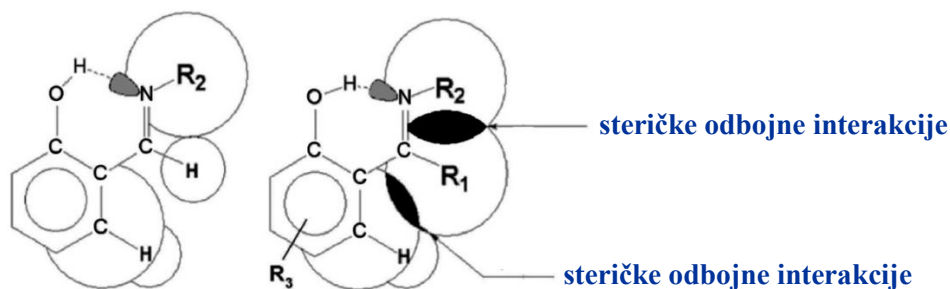
Slika 2-15. Shematski prikaz steričkih odbojnih interakcija u o -hidroksiarilnim Schiffovim bazama.
