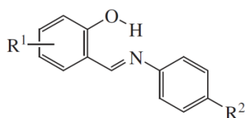
Slika 2-14. Strukture derivata Schiffove baze 11 .
