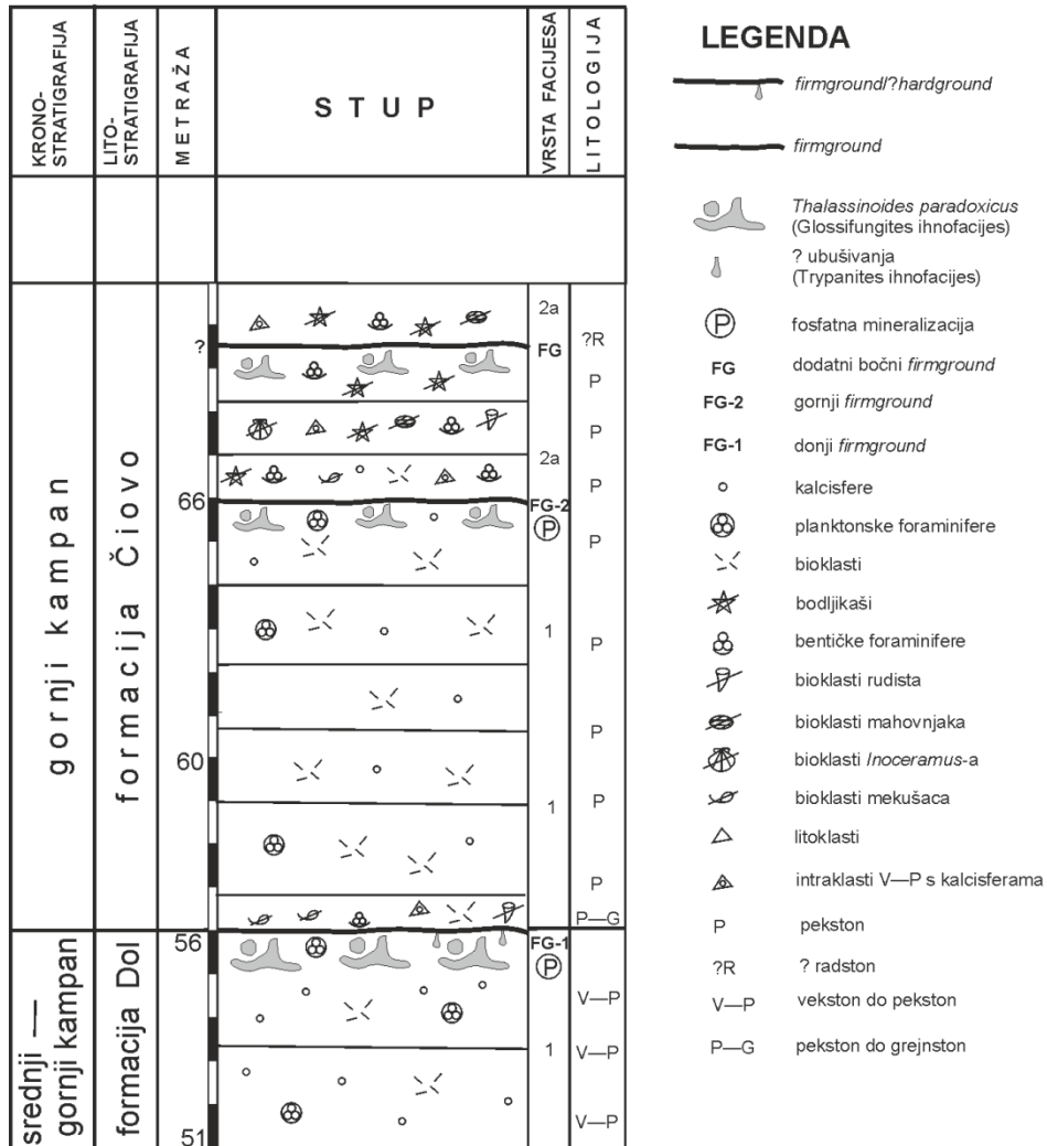
Slika 26 Detalj geološkog stupa (sl. 11) sa prikazom položaja donjeg (FG-1), gornjeg (FG-2) i dodatnog bočnog firmground-a zabilježenih u srednjo do gornjokampanskom vapnenačkom slijedu (formacije Dol i Čiovo) na otoku Čiovo, sa pripadajućom legendom.
