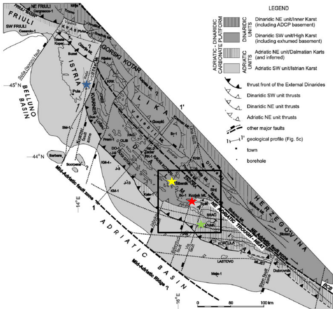
Slika 4 Pojednostavljena tektonska karta sjeveroistočne Jadranske regije koja prikazuje današnji raspored tektono-stratigrafskih jedinica koje su prepoznate na području Jadransko-Dinaridske karbonatne platforme (ADCP sensu Korbar, 2009) (preuzeto iz Korbar, 2009), s ucrtanim istraživanim lokalitetima Šibenik (žuta zvijezda), Čiovo (crvena zvijezda) i Hvar (zelena zvijezda) na području središnje Dalmacije (pravokutnik), te lokalitetom Labin-Koromačno (plava zvijezda) na području istočne Istre.
