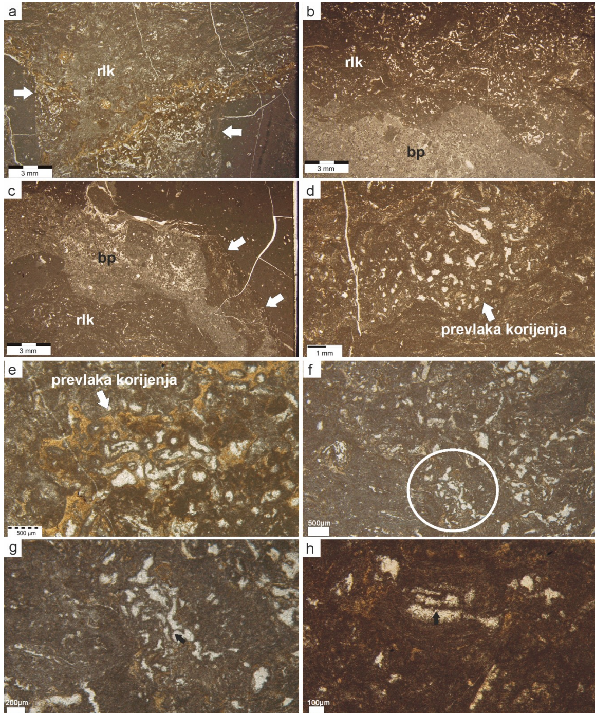
Slika 25 Mikrofotografija obilježja kompozitne površine zabilježene u formaciji Gornji Humac (lokalitet Šibenik, sl. 8, 22). a Thalassinoides u oštrm kontaktu s okolnim bioklastičnim vekstonom (bijele strelice). Bioturbacija je ispunjena s laminiranom rizogenom kalkretom (rlk). b , c Interkalacija bioklastičnog pekstona
