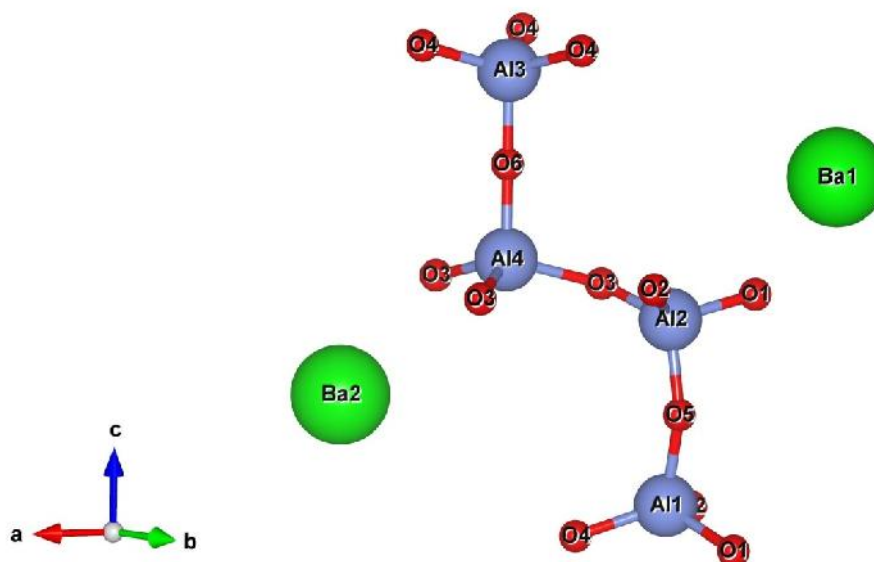
Slika 18. Shema razmjesta četiri simetrijski neekvivalentna atoma aluminija i atoma barija u strukturi niskotemperaturne faze \text{BaAl}_2\text{O}_4 . Nacrtano prema atomskim položajima iz literature 16 .
