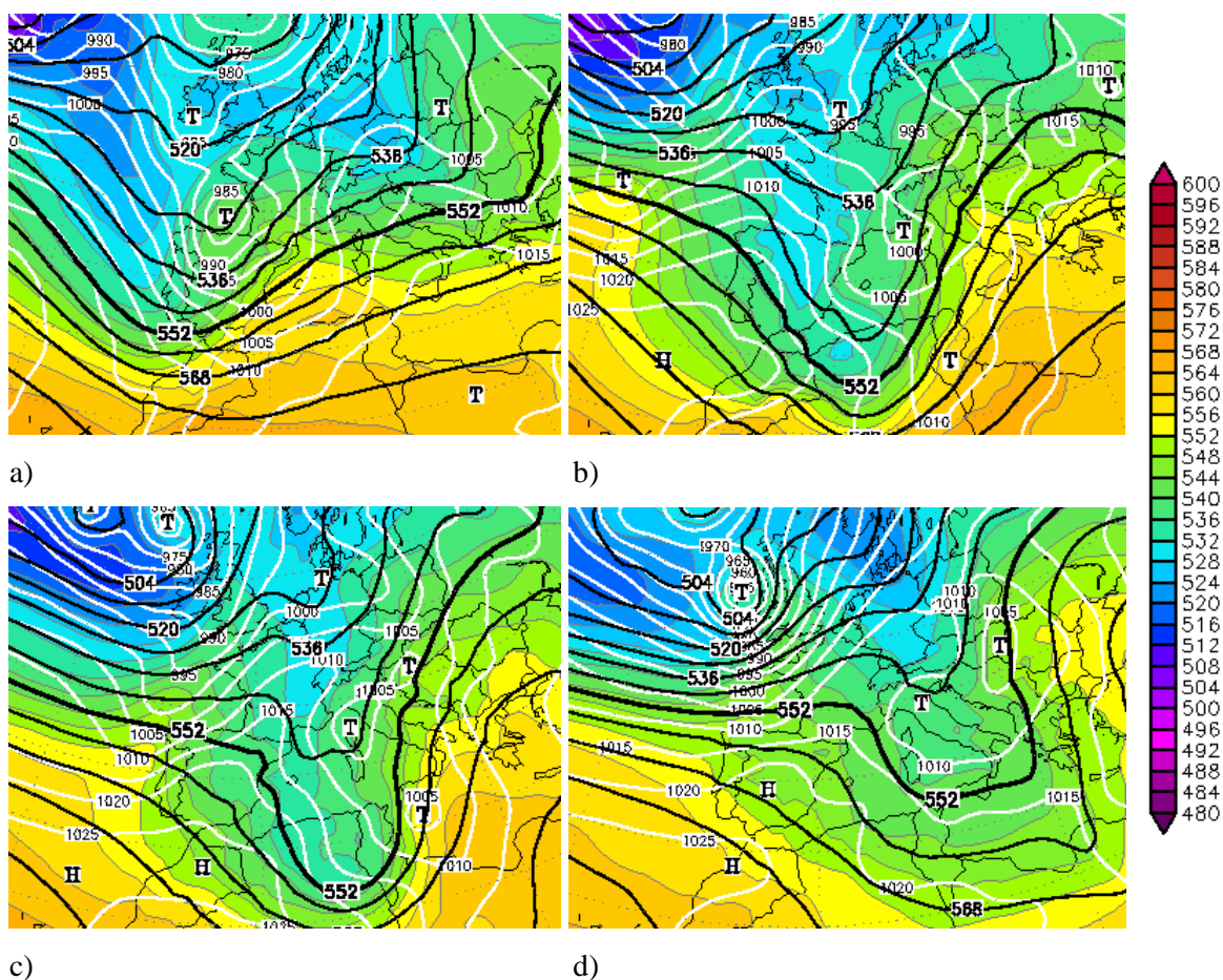
Slika 33. Polje geopotencijala 500 hPa plohe (gdam, crno), prizemnog tlaka (hPa, bijelo) i relativne topografije RT 500/1000 hPa (gdam, obojeno) za 10. veljače 2014. u 00 UTC (a) i u 18 UTC (b), za 11. veljače 2014. u 06 UTC (c) i za 12. veljače u 12 UTC (d)
