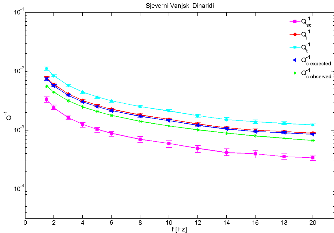
Slika A.18 Rezultati za sjeverne Vanjske Dinaride. Q^{-1} -faktori u ovisnosti o frekvenciji dobiveni MLTWA metodom te mjereni Q_c^{-1} preuzet iz Dasović (2015). Prikazane su i pripadajuće standardne devijacije dobivene za parove Le^{-1} i B_0 područja 68% pouzdanosti F-distribucije.
