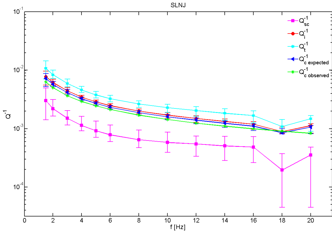
Slika A.15 Rezultati za postaju SLNJ. Q^{-1} -faktori u ovisnosti o frekvenciji dobiveni MLTWA metodom te mjereni Q_c^{-1} observed preuzet iz Dasović (2015). Prikazane su i pripadajuće standardne devijacije dobivene za parove Le^{-1} i B_0 područja 68% pouzdanosti F-distribucije.
