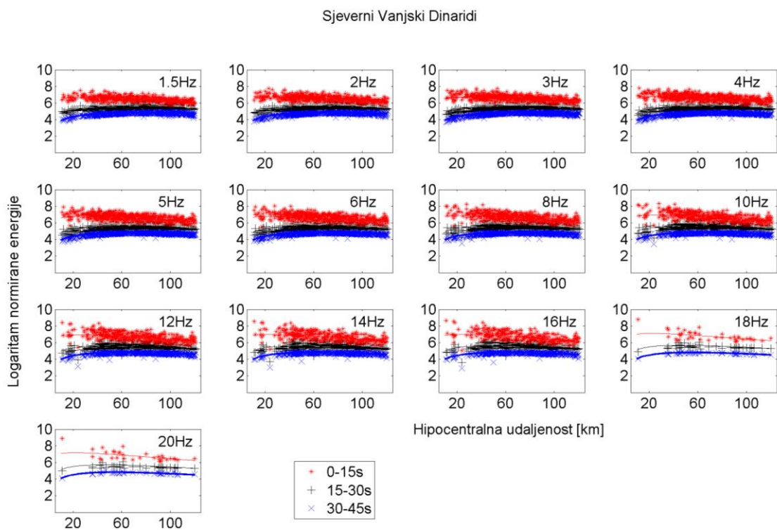
Slika A.6 Rezultati za sjeverne Vanjske Dinaride. Izmjerene energije seizmograma, u tri vremenska prozora: 0–15 s(*), 15–30 s (+), 30–45 s (x), zajedno s teorijskim krivuljama energije koje predstavljaju najbolju prilagodbu mjerenjima, u ovisnosti o hipocentralnoj udaljenosti.
