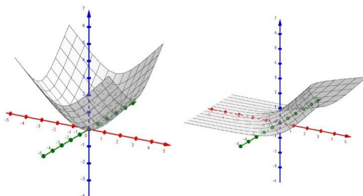
Slika 3.5: Plohe (3.11) i (3.12) za a = 1
