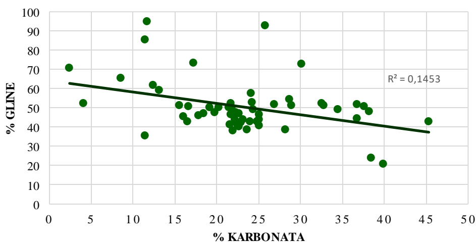
Slika 19 Grafikon obrnuto proporcionalnog odnosa karbonatne i glinene komponente u 58 analiziranih uzoraka sedimenta duboke jezgre iz delte rijeke Mirne
