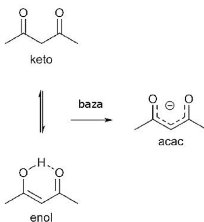
Slika 4. Keto-enolna ravnoteža acetilacetona i nastajanje acetilacetonatnog aniona 9
