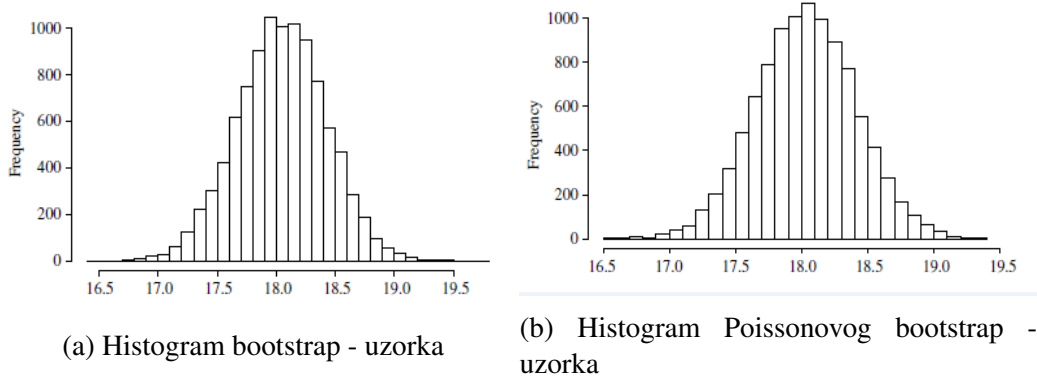
Slika 4.8: Histogrami
