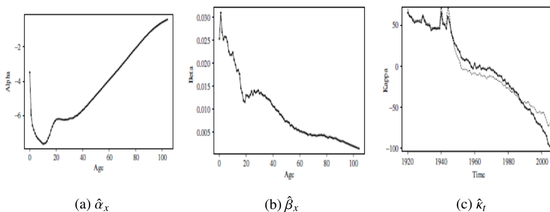
Slika 4.4: Procijenjeni parametri
