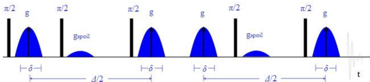
Slika 2.9.1. Shematski prikaz pulsne sekvence PGDSTE. U shemi su označeni puls od 90^\circ ( \pi/2 ), gradijent (g), vrijeme akvizicije (t), spoil gradijent ( g_{\text{spoil}} ), vrijeme trajanja gradijenta ( \delta ) i polovina vremena difuzije ( \Delta/2 ). 15
