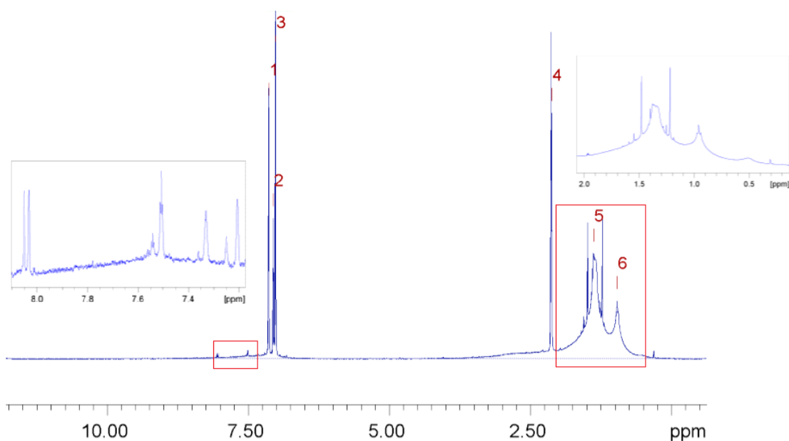
Slika 4.1.1. Reprezentativni spektar ^1\text{H} NMR uzorka S10 ( \gamma = 20,54 \text{ g L}^{-1} ) snimljen u deuteriranom otapalu toluen- \text{d}_8 pri 25 °C.
