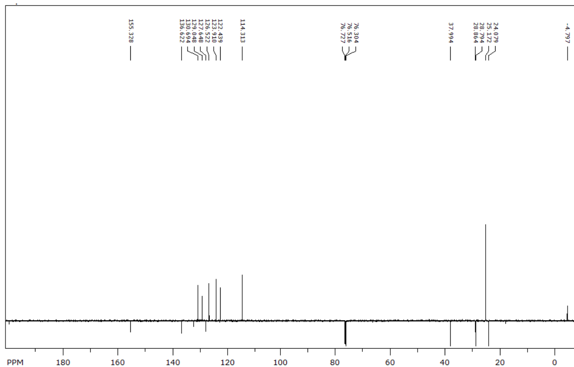
D1.4. 13 C NMR spektar spoja 3
