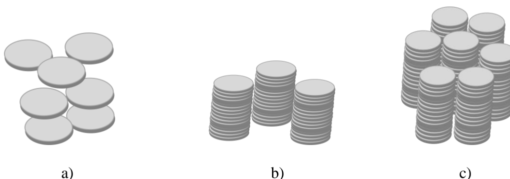
Slika 15. Struktura a) diskoliki nematik, b) kolonska nematička faza, c) heksagonalna kolonska faza 7
