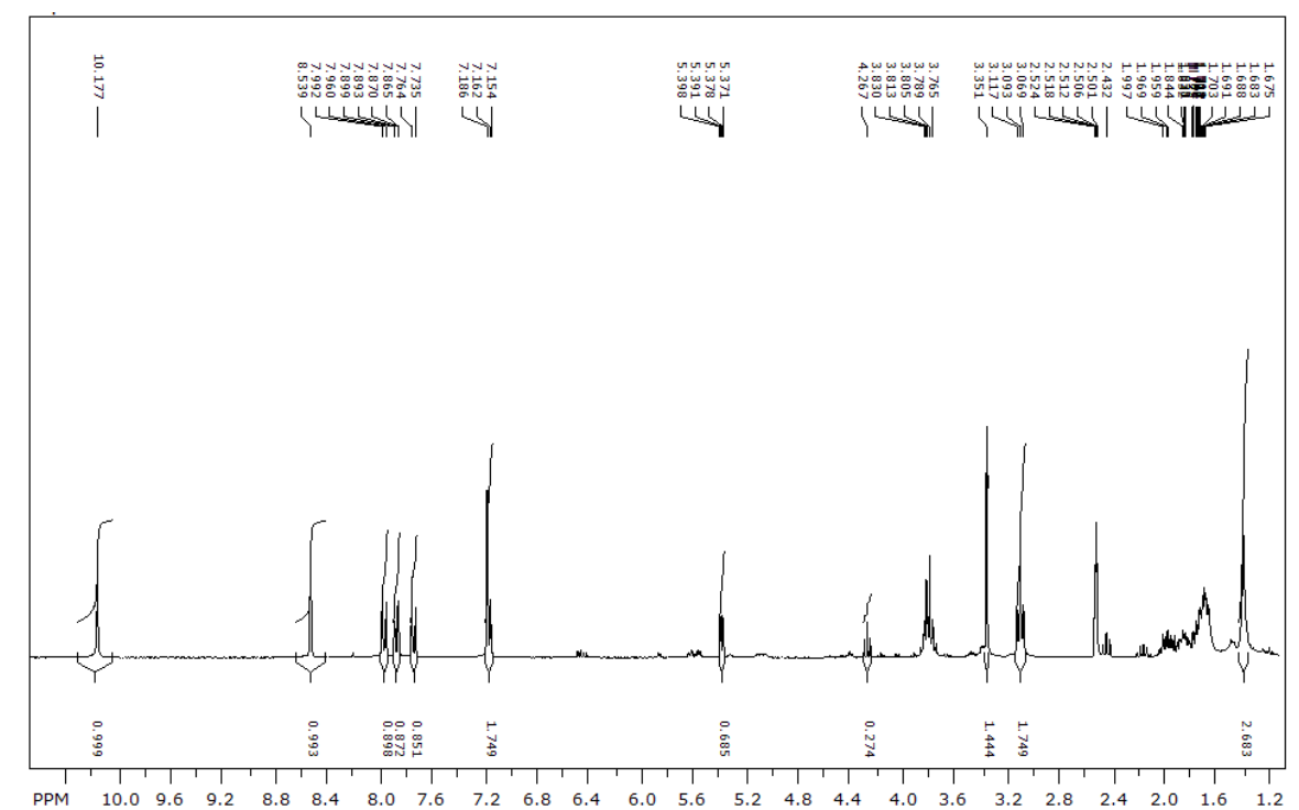
D1.5. 1 H NMR spektar spoja 4
