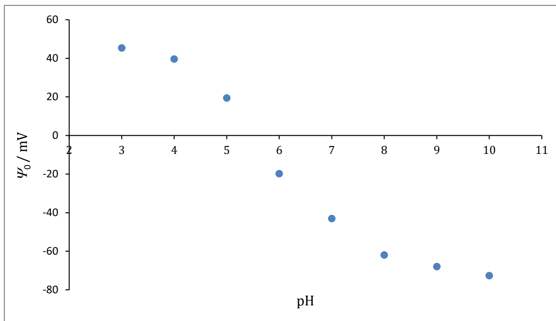
Slika 22. Ovisnost površinskog potencijala cerijevog oksida o pH vrijednosti otopine HCl ( c = 0,001 \text{ mol dm}^{-3} ) i NaCl ( c = 0,001 \text{ mol dm}^{-3} ) uz pretpostavljen stalan kapacitet pločastog kondenzatora ( C = 1,7 \text{ F m}^{-2} ), l = 20 \text{ Å} , \theta = 25 \text{ °C} .
