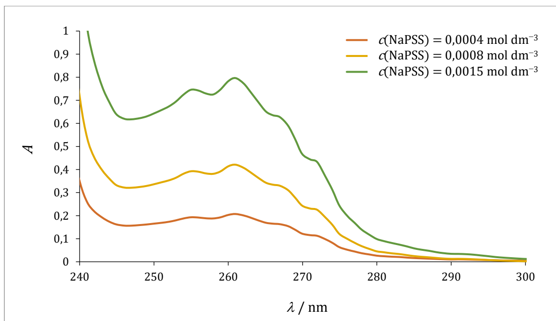
Slika 29. Koncentracijska ovisnost spektra vodene otopine NaPSS, HCl ( c = 0,001 \text{ mol dm}^{-3} ), NaCl ( c = 0,001 \text{ mol dm}^{-3} ), l = 1 cm, \theta = 25 °C.
