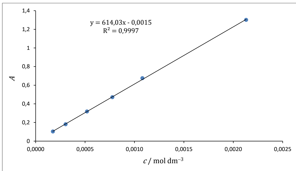
Slika 28. Koncentracijska ovisnost apsorbancije vodene otopine NaPSS, \lambda = 261 nm, l = 1 cm, \theta = 25 °C.
