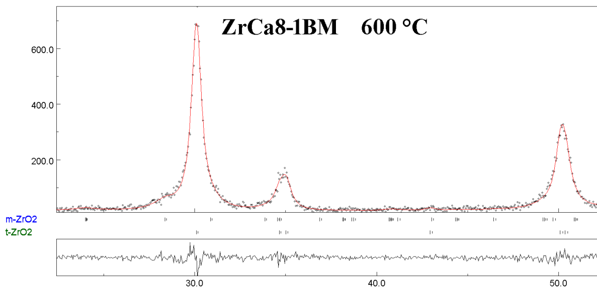
Slika D56. Rezultat Rietveldovog utočnjavanja difraktograma uzorka ZrCa8-1BM žarenog na 600°C. Razlika izračunatog i dobivenog difraktograma prikazana je u donjem pravokutniku.
