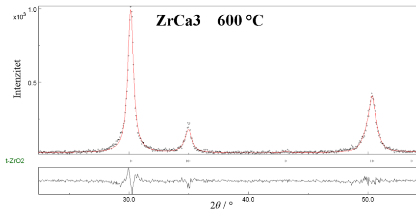
Slika D10. Rezultat Rietveldovog utočnjavanja difraktograma uzorka \text{ZrCa}_3 žarenog na 600\text{ }^\circ\text{C} . Razlika izračunatog i dobivenog difraktograma prikazana je u donjem pravokutniku.
