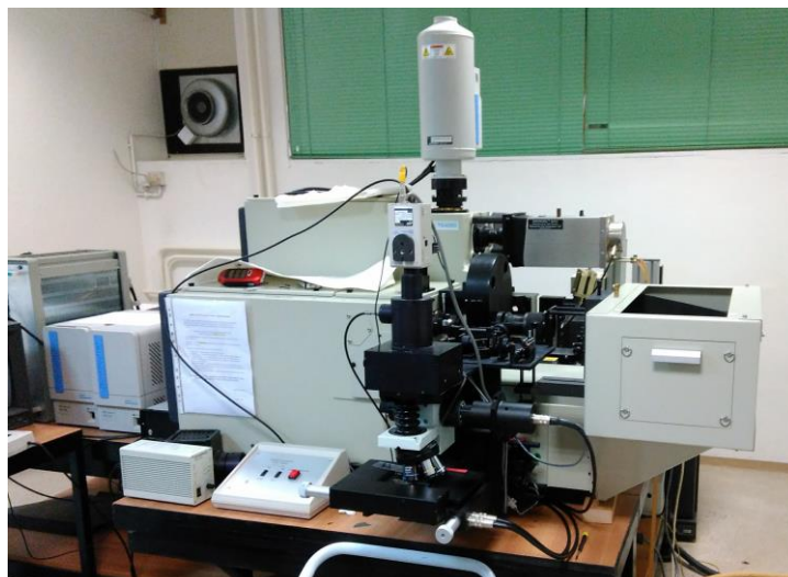
3.9. Horiba T64000 Ramanov spektrometar.
