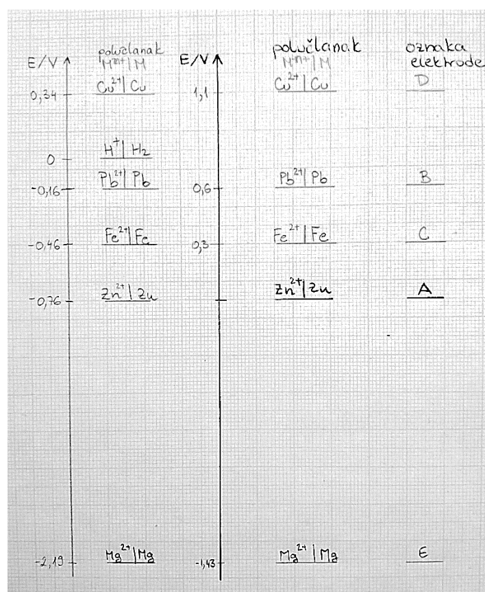
Slika 9. Jednodimenzijski dijagram relativnih redukcijskih potencijala prema tablici 3. i Koraku 8.
