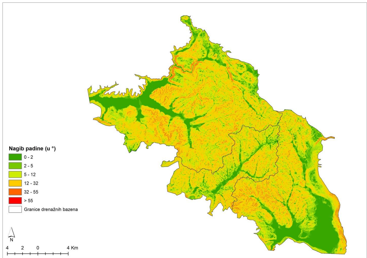
Slika 7: Nagib padina
