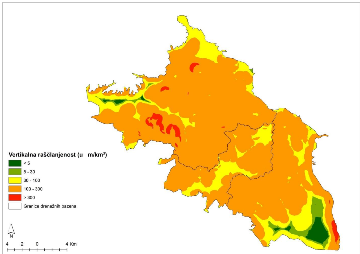
Slika 9: Vertikalna raščlanjenost
