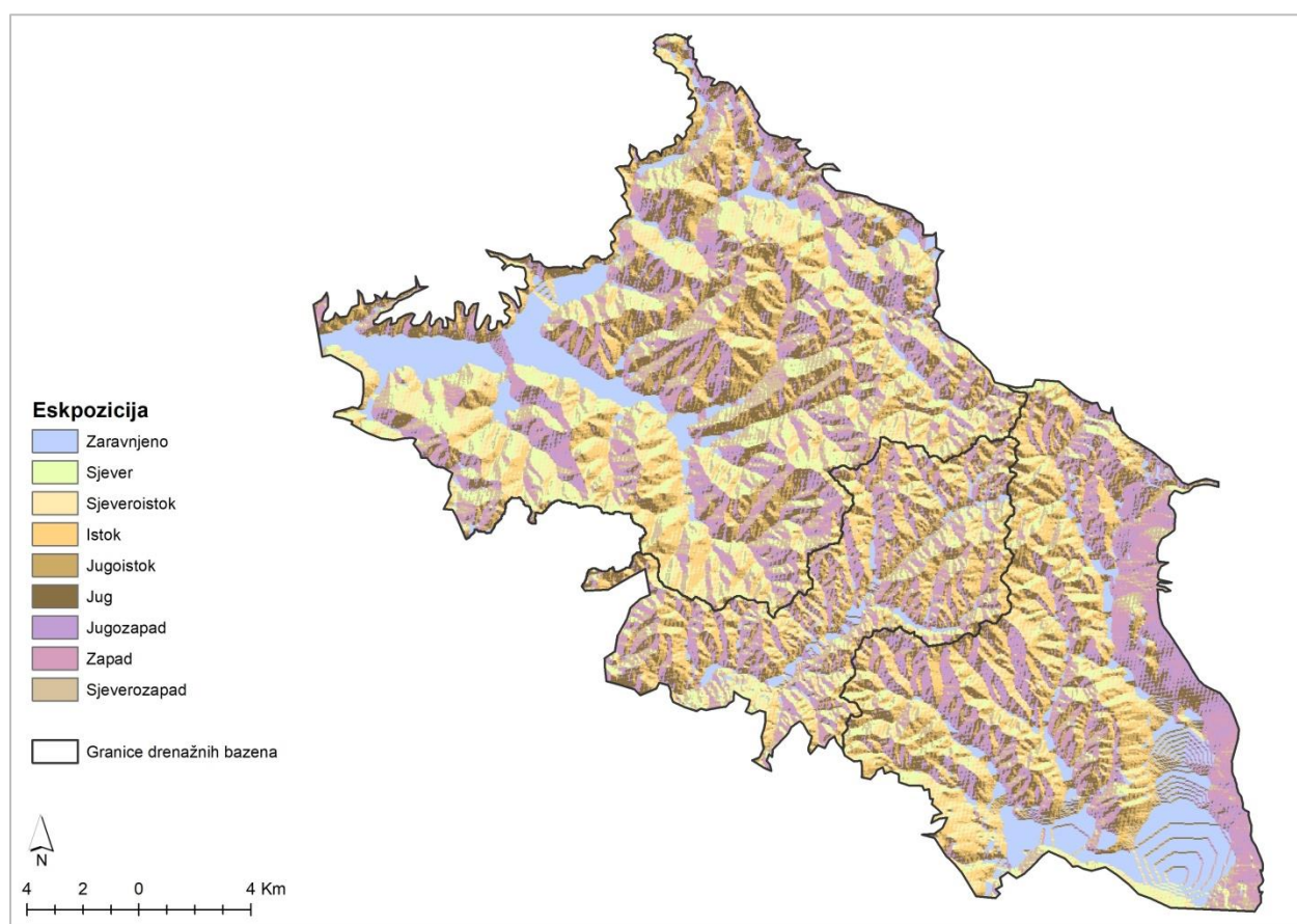
Slika 11: Ekspozicija padina
