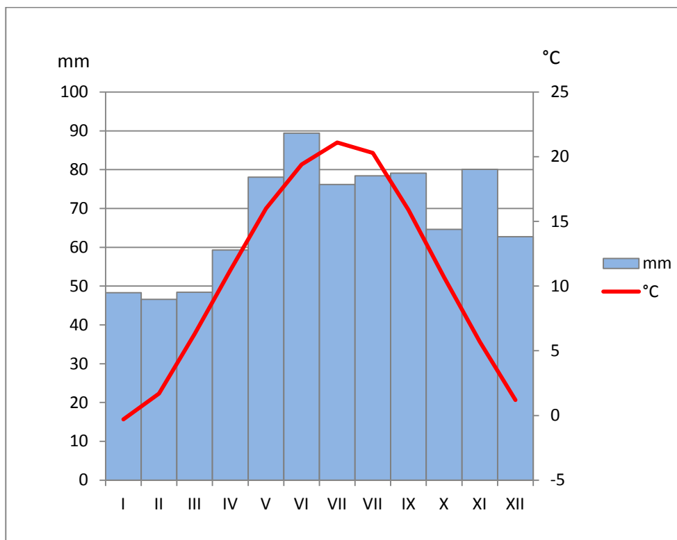
Sl. 3. Srednje mjesečne vrijednosti temperature i padalina u Bjelovaru za razdoblje 1949.-2015.
