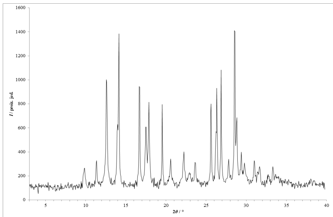
Slika 82 – Rentgenski difraktogram praškastog uzorka dobivenog kristalizacijom iz otopine lam i nia u etil-acetatu.
