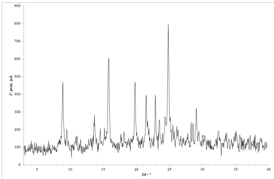
Slika 115 – Rentgenski difraktogram praškastog uzorka dobivenog ručnom mehanokemijskom sintezom fizičke smjese lam i van s dodatkom katalitičke količine 1,2-dimetoksietana.
