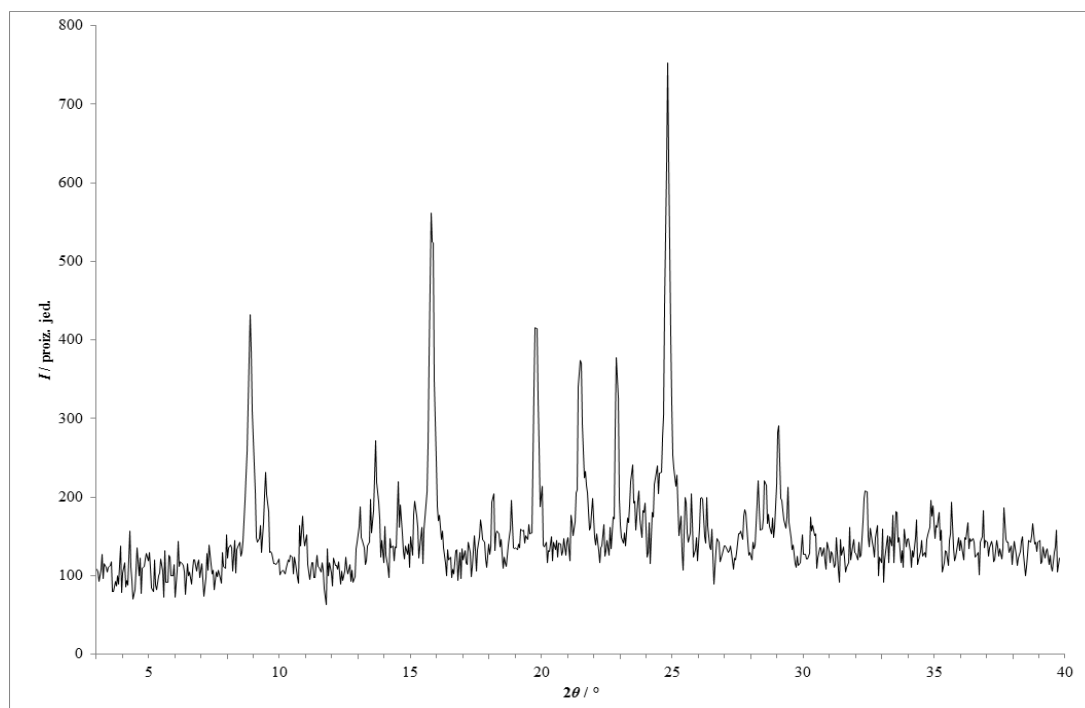
Slika 181 – Rentgenski difraktogram praškastog uzorka dobivenog mehanokemijskom sintezom u mlinu fizičke smjese lam i van s dodatkom katalitičke količine butil-acetata.
