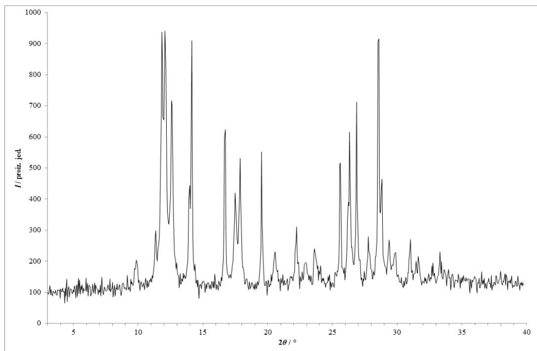
Slika 129 – Rentgenski difraktogram praškastog uzorka dobivenog ručnom mehanokemijskom sintezom fizičke smjese lam i kaf s dodatkom katalitičke količine 1-butanola.
