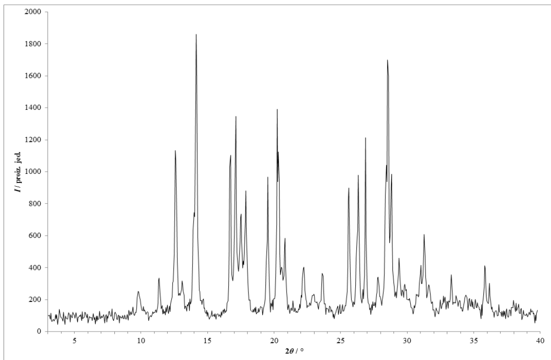
Slika 269 – Rentgenski difraktogram praškastog uzorka dobivenog statičkom kompresijom fizičke smjese lam i fru tlakom od 750 MPa s dodatkom katalitičke količine acetonitrila.
