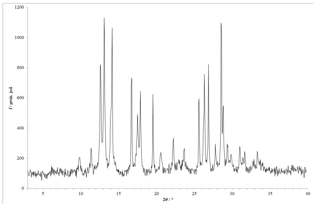
Slika 243 – Rentgenski difraktogram praškastog uzorka dobivenog statičkom kompresijom fizičke smjese lam i van tlakom od 750 MPa s dodatkom katalitičke količine toluena.
