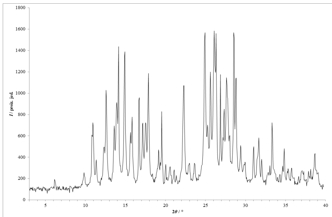
Slika 265 – Rentgenski difraktogram praškastog uzorka dobivenog statičkom kompresijom fizičke smjese lam i nia tlakom od 750 MPa s dodatkom katalitičke količine vode.
