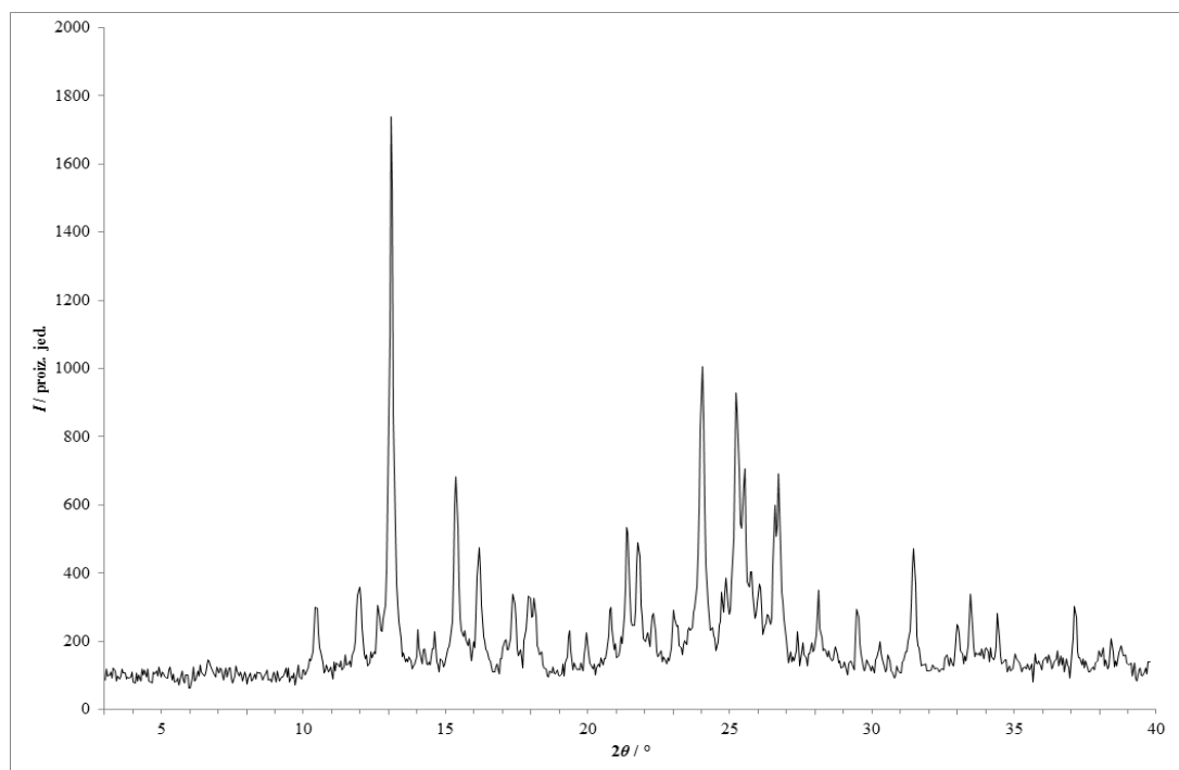
Slika 44 – Rentgenski difraktogram praškastog uzorka dobivenog kristalizacijom iz otopine lam i van u 1-butanolu.
