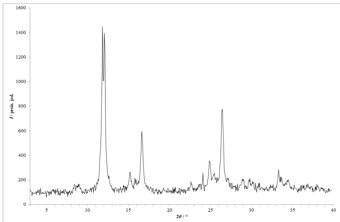
Slika 58 – Rentgenski difraktogram praškastog uzorka dobivenog kristalizacijom iz otopine lam i kaf u acetonitrilu.
