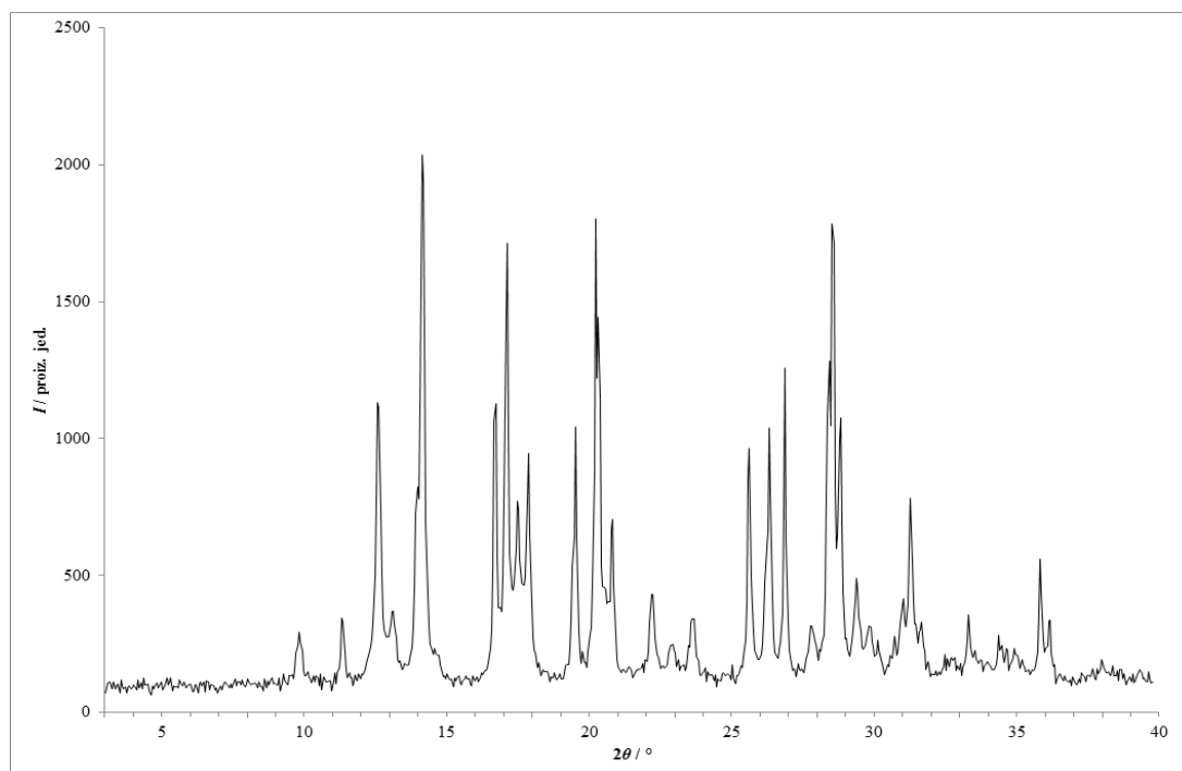
Slika 173 – Rentgenski difraktogram praškastog uzorka dobivenog ručnom mehanokemijskom sintezom fizičke smjese lam i fru s dodatkom katalitičke količine toluena.
