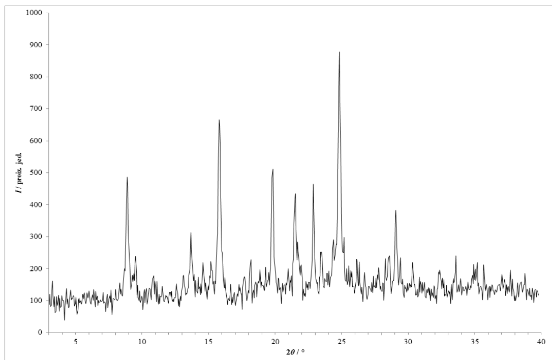
Slika 179 – Rentgenski difraktogram praškastog uzorka dobivenog mehanokemijskom sintezom u mlinu fizičke smjese lam i van s dodatkom katalitičke količine anisola.
