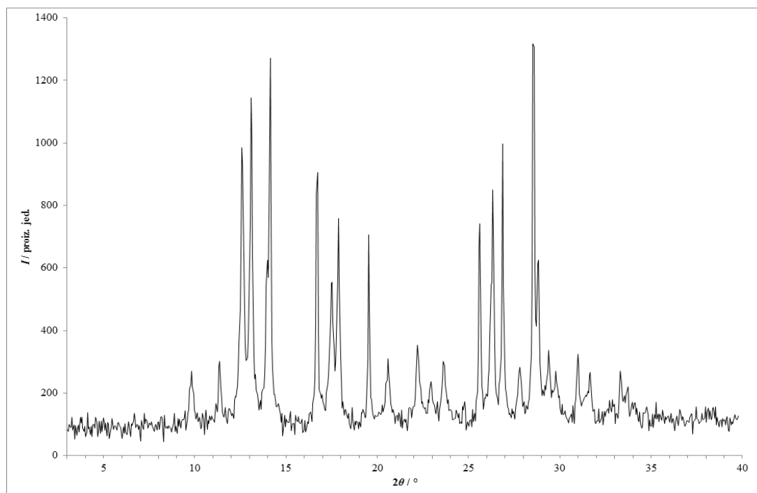
Slika 303 – Rentgenski difraktogram praškastog uzorka dobivenog brzom udarnom kompresijom fizičke smjese lam i van pri tlaku pneumatske posude od 9 bar.
