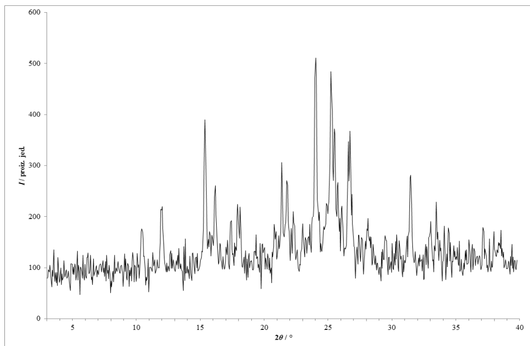
Slika 76 – Rentgenski difraktogram praškastog uzorka dobivenog kristalizacijom iz otopine lam i nia u 1-butanolu.
