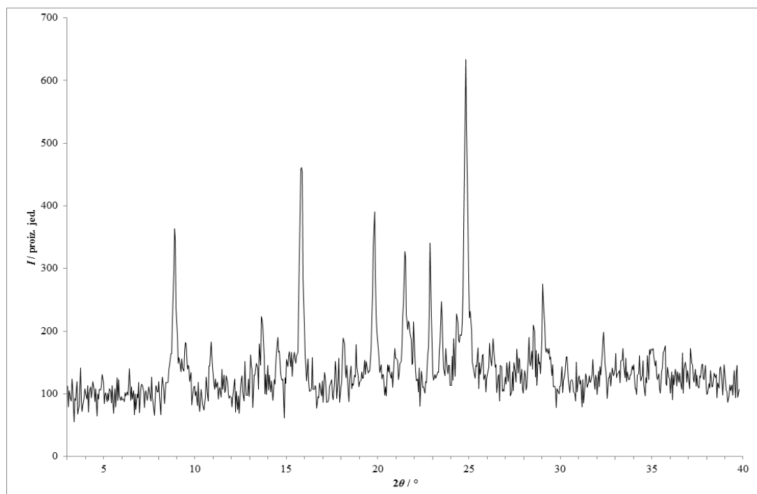
Slika 45 – Rentgenski difraktogram praškastog uzorka dobivenog kristalizacijom iz otopine lam i van u butil-acetatu.
