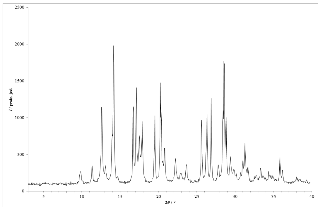
Slika 227 – Rentgenski difraktogram praškastog uzorka dobivenog mehanokemijskom sintezom u mlinu fizičke smjese lam i fru s dodatkom katalitičke količine kloroforma.
