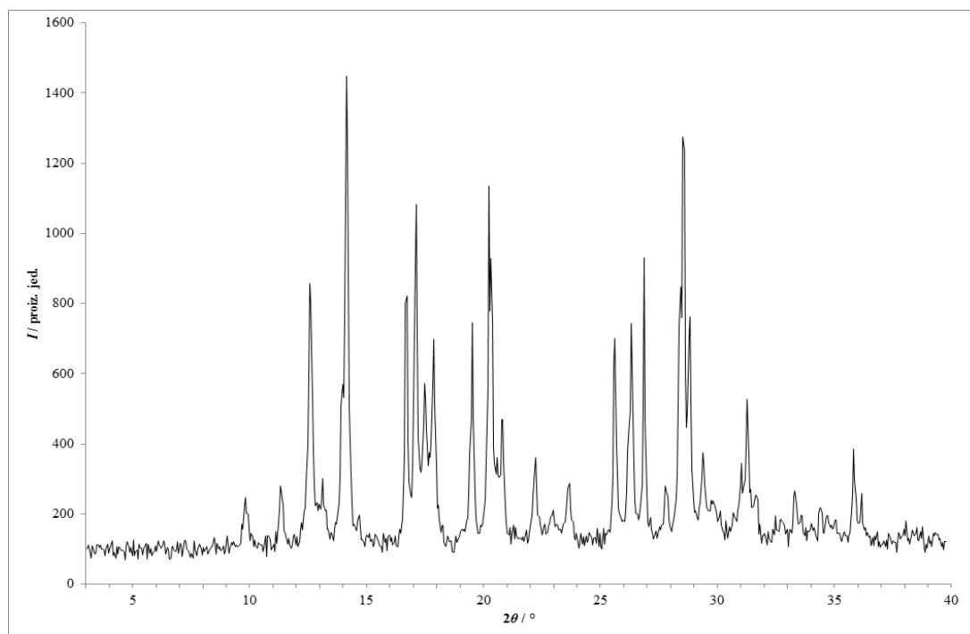
Slika 169 – Rentgenski difraktogram praškastog uzorka dobivenog ručnom mehanokemijskom sintezom fizičke smjese lam i fru s dodatkom katalitičke količine etil-acetata.
