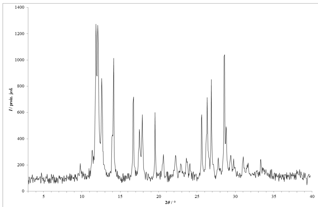
Slika 137 – Rentgenski difraktogram praškastog uzorka dobivenog ručnom mehanokemijskom sintezom fizičke smjese lam i kaf s dodatkom katalitičke količine metil- tert -butil-etera.
