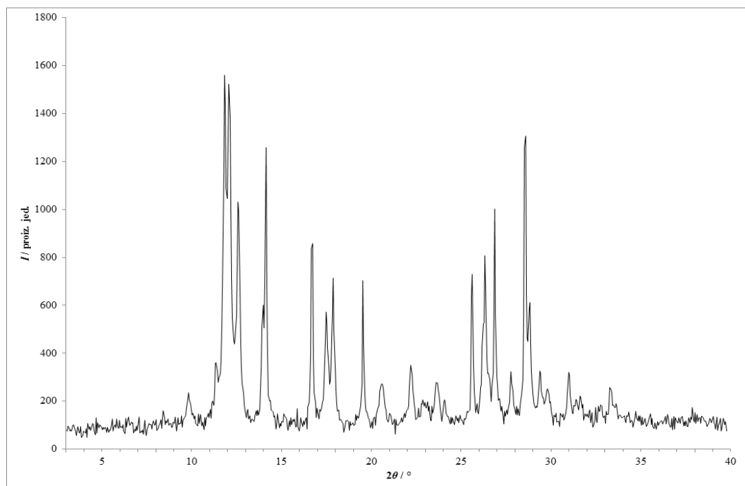
Slika 197 – Rentgenski difraktogram praškastog uzorka dobivenog mehanokemijskom sintezom u mlinu fizičke smjese lam i kaf s dodatkom katalitičke količine kloroforma.
