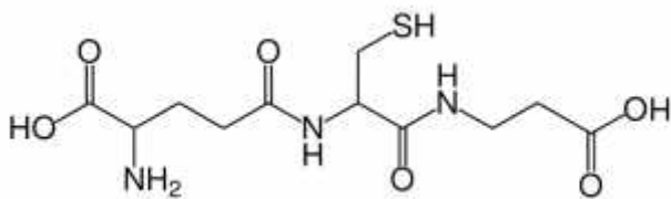
Slika 5. Strukturna formula hGSH.
