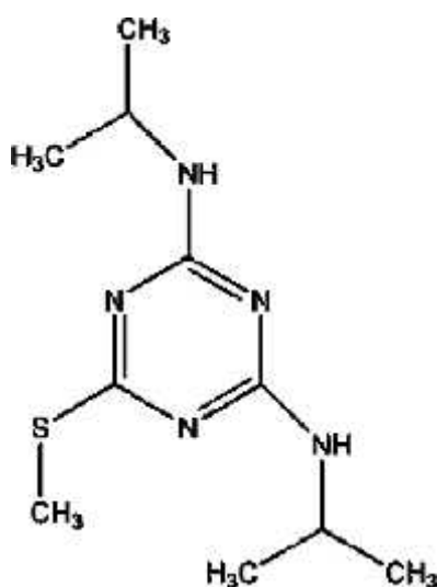
Slika 2. Strukturna formula prometrina
