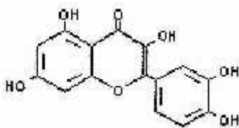
Slika 5. Kvercetin
