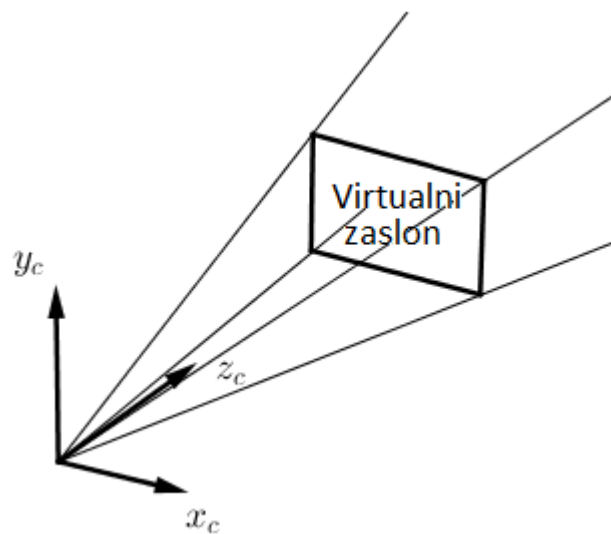
Slika 3.9: Osi kamere
