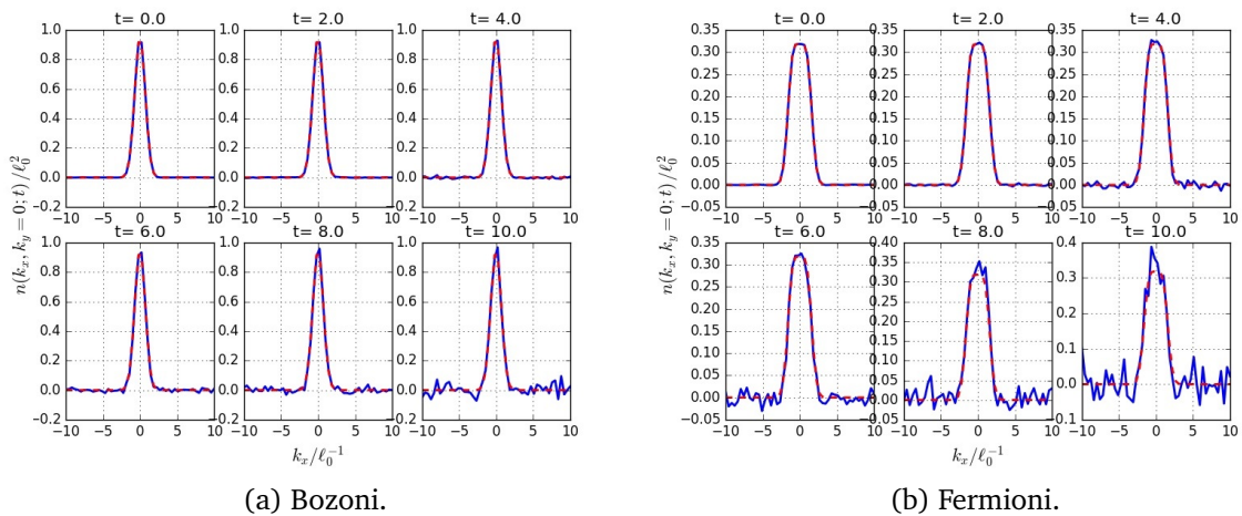
Slika 5.7: Vremenska evolucija raspodjele impulsa. Puna plava linija predstavlja numeričke rezultate, a crtkana crvena analitičke.
