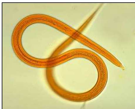
Slika 21. Nematoda.
