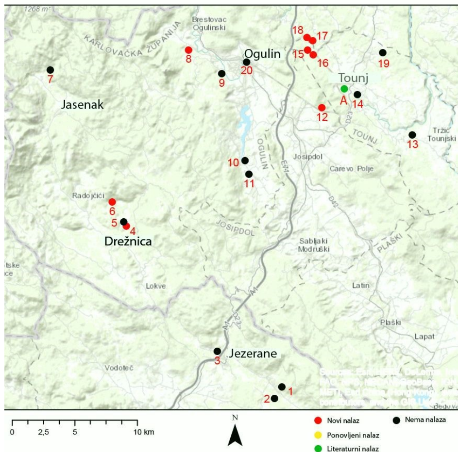
Slika 18. Karta rasprostranjenosti vrste Belgrandiella pageti
