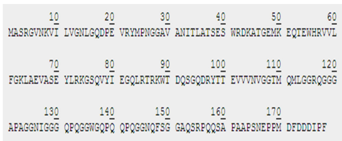
Slika 6. Slijed aminokiselina proteina SSB bakterije E. coli (izvor: UniProtKB/Swiss-Prot Protein Knowledgebase)
