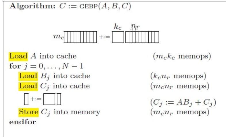
Slika 4.4: Osnovna implementacija GEBP-a
