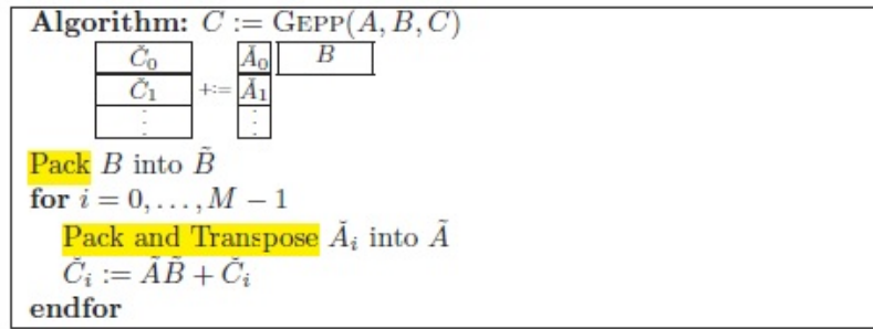
Slika 4.6: Optimizirana implementacija GEPP (individualna operacija umnoška ploča-ploča C := A_j B_j + C )
