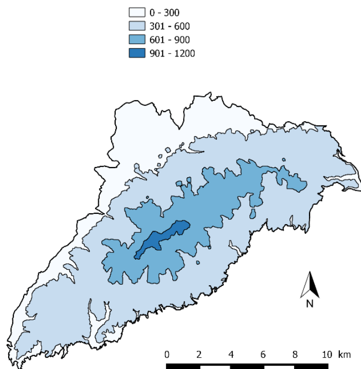
Slika 6. Raspodjela nadmorskih visina izraženih u metrima (izvor: http://geoportal.dgu.hr/wms ).
