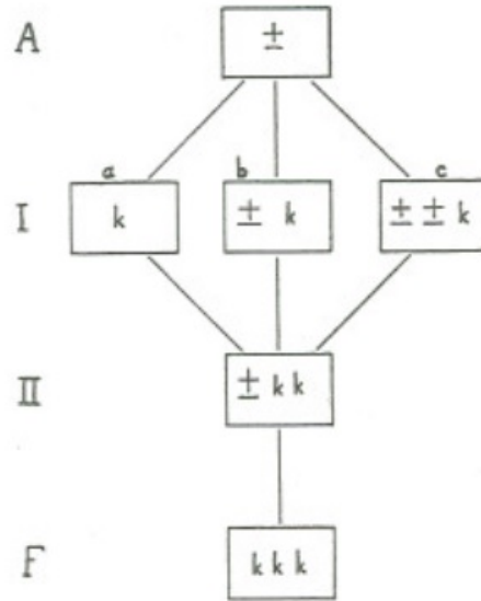
Slika 4.4: Dijagram mogućih tranzicija koje rezultiraju anihilacijom para elektron-pozitron u tri fotona. [12]
