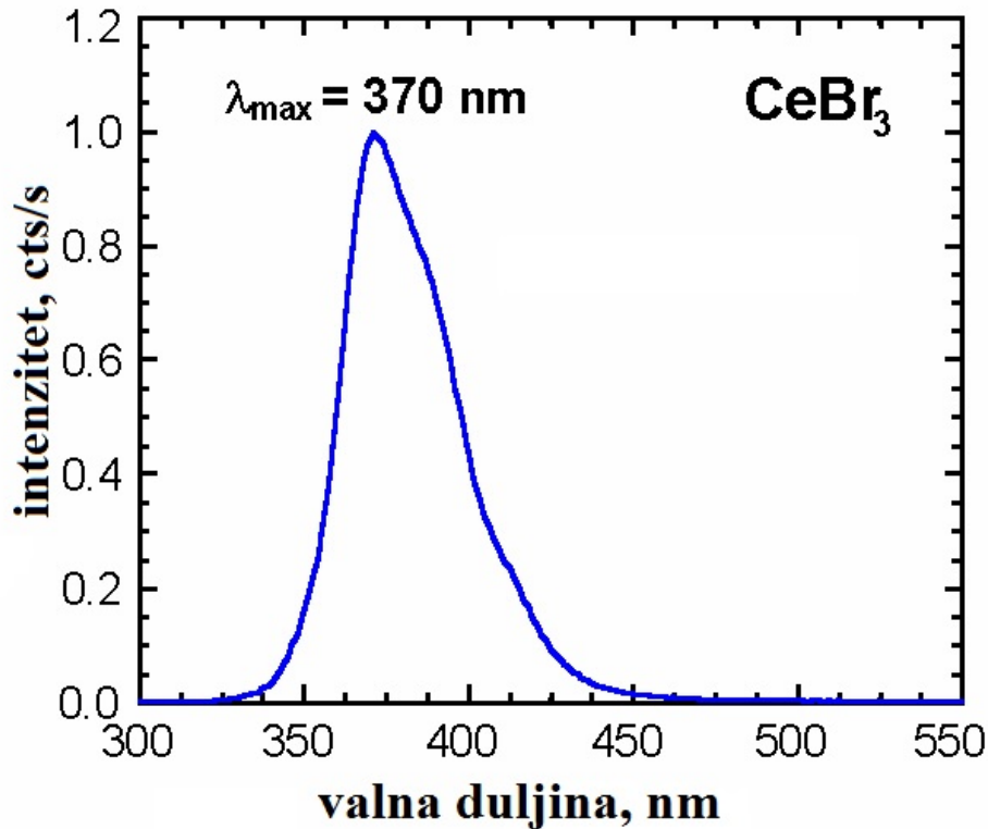
Slika 6.3: Spektar optičke emisije \text{CeBr}_3 detektora nastala izlaganjem X - zračenju. [16]
