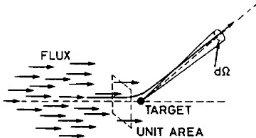
Slika 2.6: Grafički prikaz raspršenja snopa čestica I na metu. [2]
