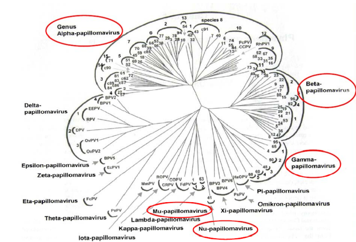
Slika 1. Klasifikacija HPV virusa. Preuzeto s Ethel-Mischele de Villiers i sur. (2004).
