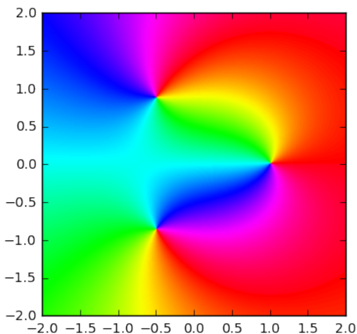
Slika 2.7: Fazni portret
